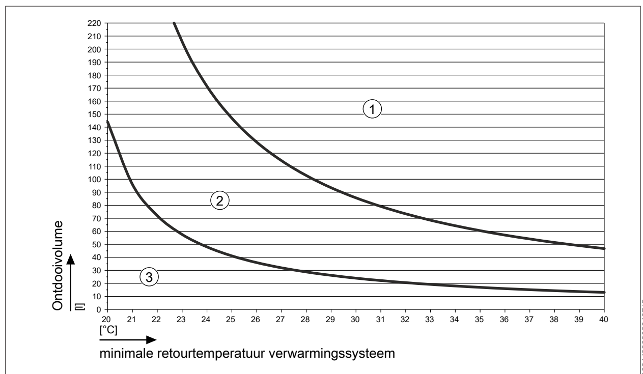
Afb. 2: CHA-16/20
