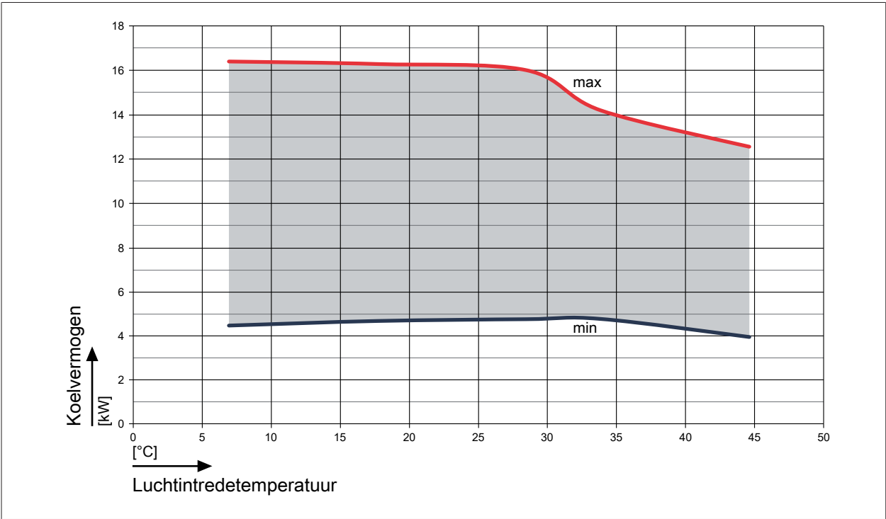
Afb. 9: Koelvermogen bij een aanvoer van 7 °C
