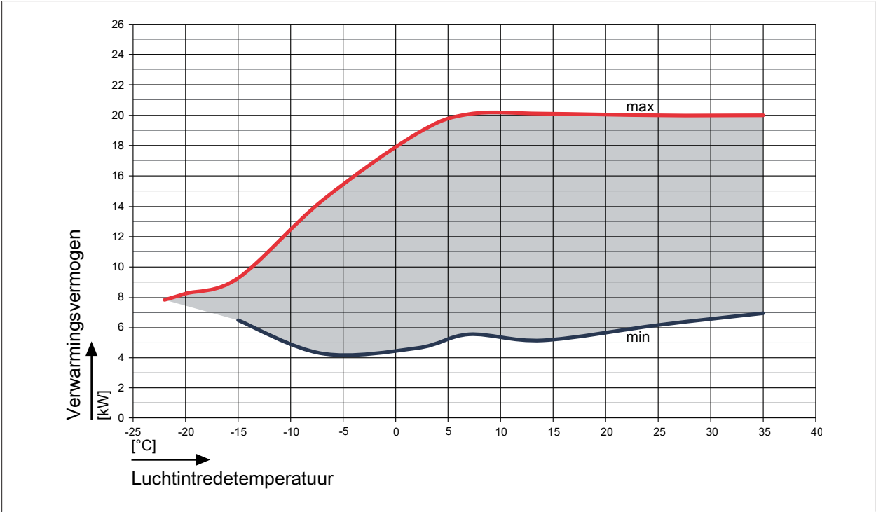
Afb. 7: Verwarmingsvermogen bij een aanvoer van 65 °C
