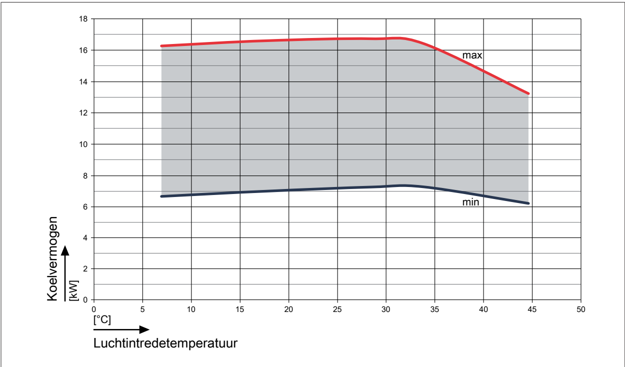
Afb. 8: Koelvermogen bij een aanvoer van 18 °C
