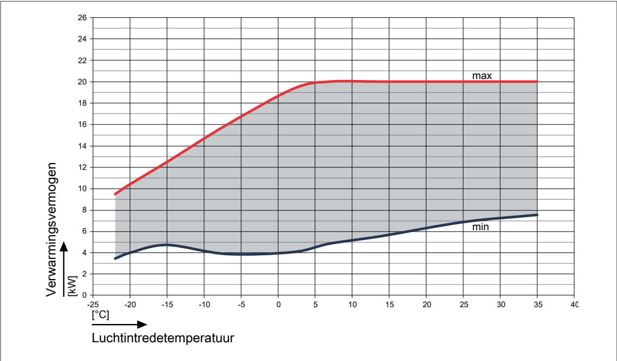
Afb. 6: Verwarmingsvermogen bij een aanvoer van 55 °C
