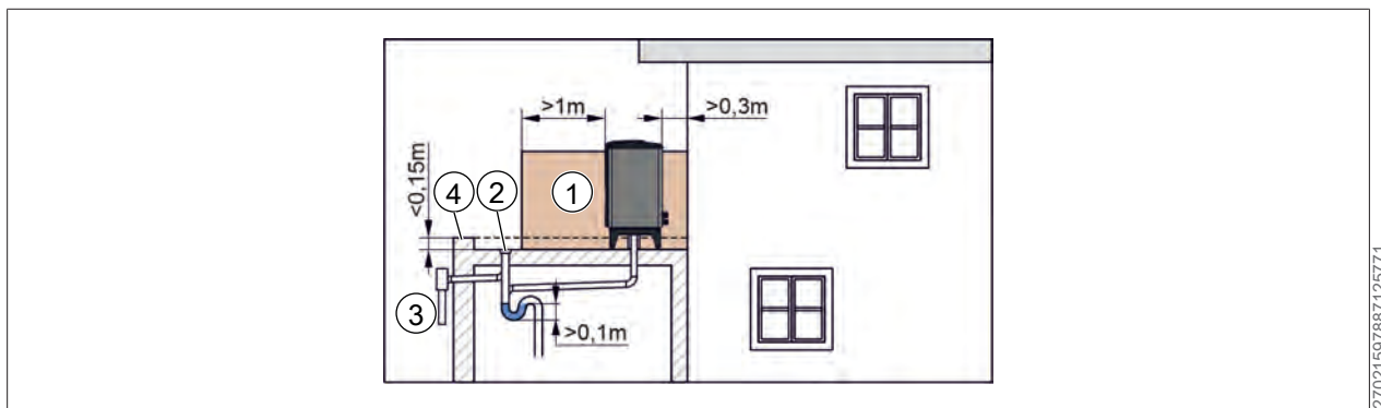
1 Veiligheidszone
