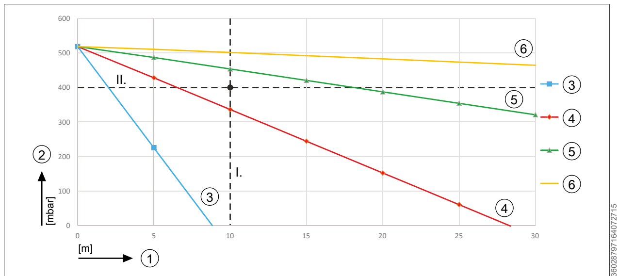
Afb. 1: PREMIUM CHA-16/20 Beschikbare opvoerhoogten
