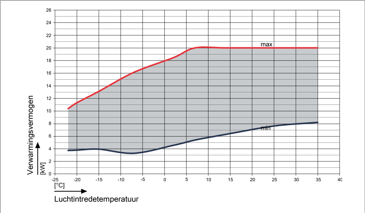
Afb. 5: Verwarmingsvermogen bij een aanvoer van 45 °C
