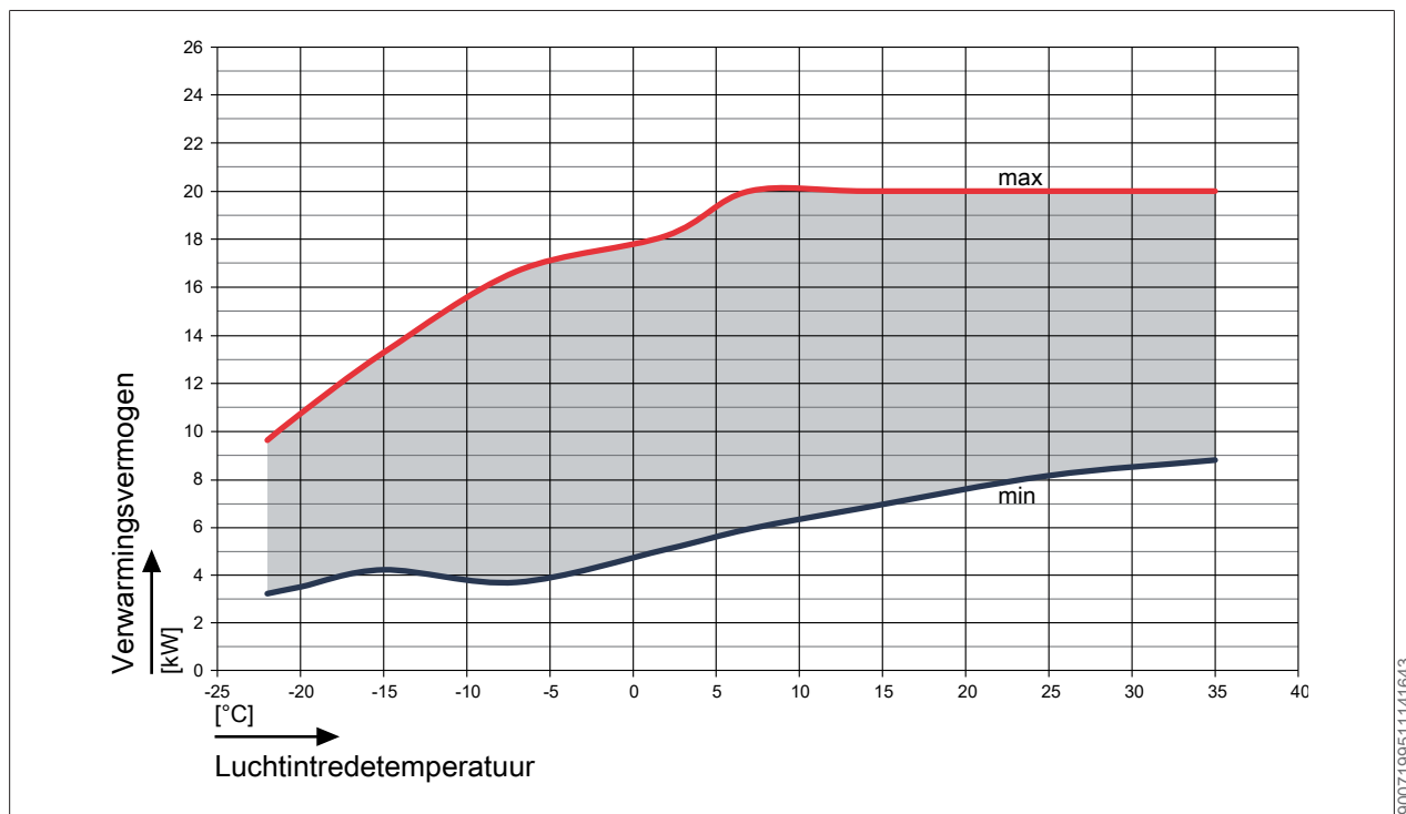
Afb. 4: Verwarmingsvermogen bij een aanvoer van 35 °C
