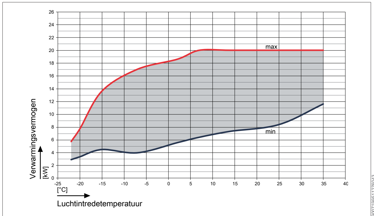
Afb. 3: Verwarmingsvermogen bij een aanvoer van 25 °C
