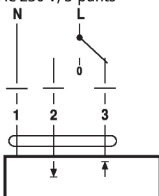
Aansluitschema's AC 230 V, 3-punts
