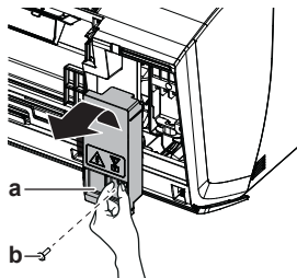
a Servicedeksel b Schroef servicedeksel
