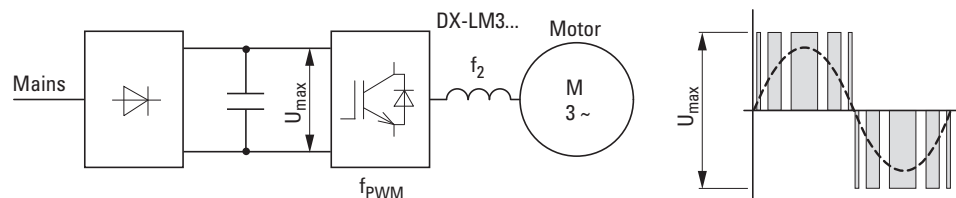
Abbildung 32: Bemessungsdaten DX-LM3...:
