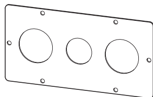
Abbildung 10: Abdeckplatte mit Löchern für Kabelverschraubungen (FS4, FS5)
