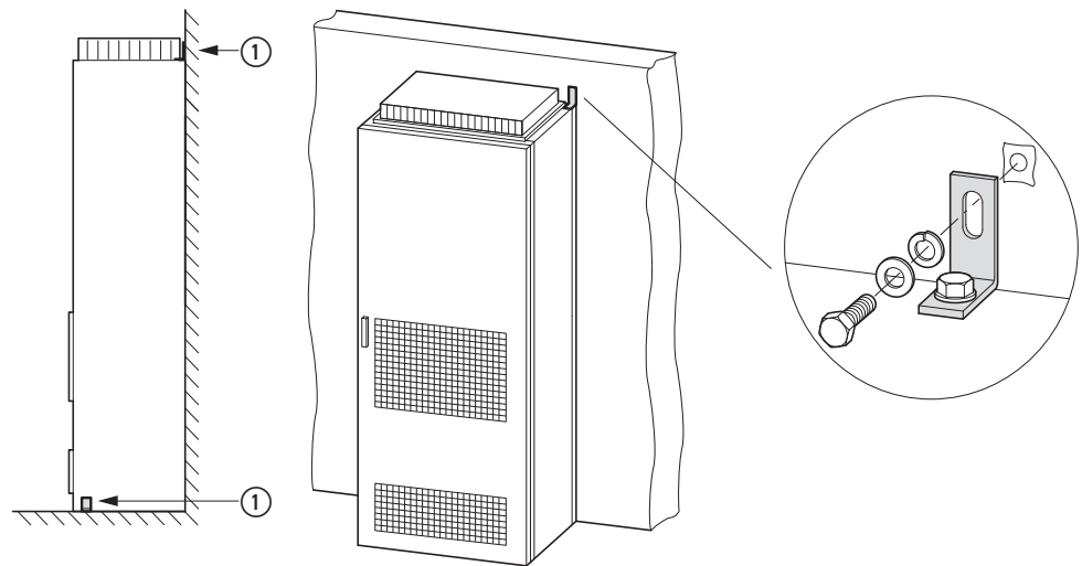
Abbildung 49: Standsichere Schaltschrankaufstellung
