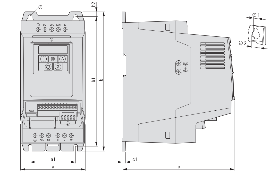
Abbildung 92: Baugrößen FS2, FS3, FS4 und FS5 in IP20 (NEMA 0)
