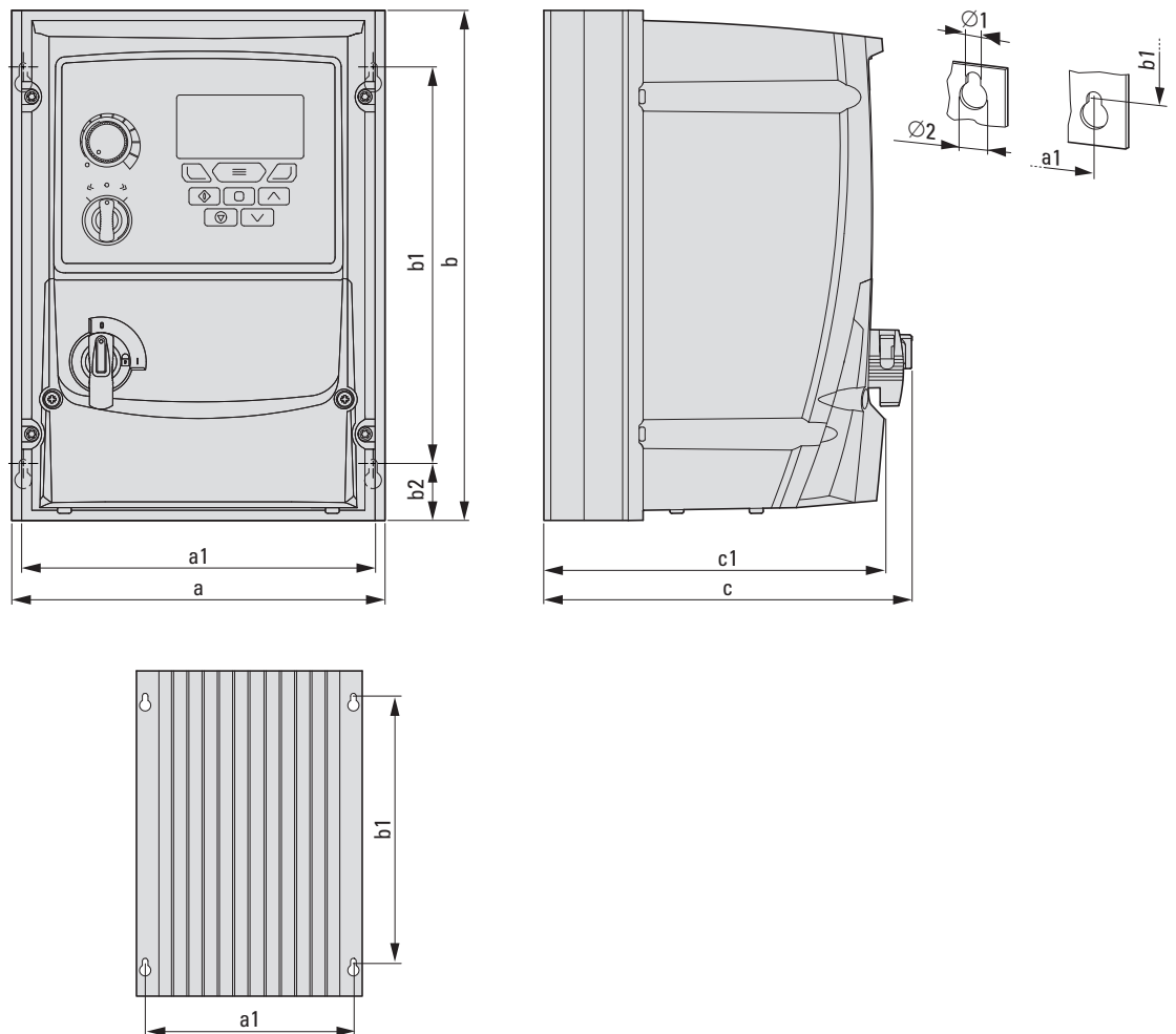
Abbildung 94: Baugrößen FS2, FS3 und FS4 in IP66 (NEMA 4X)
