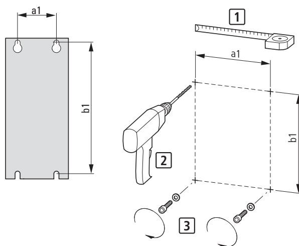
Abbildung 45: Montagemaße
