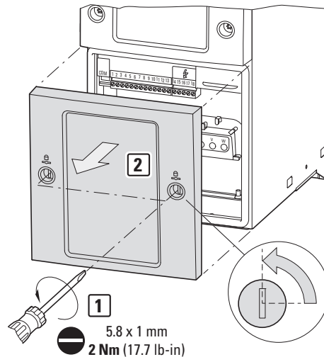
Abbildung 60: Deckel entfernen
