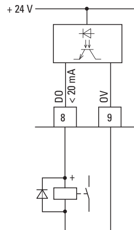
Abbildung 82: Anschlussbeispiel (Koppelrelais mit Freilaufdiode: ETS4-VS3; Artikel-Nr. 083094)
