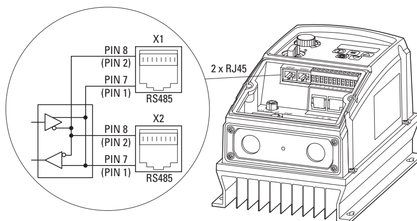
Abbildung 85: RJ45-Schnittstellen (IP66)
