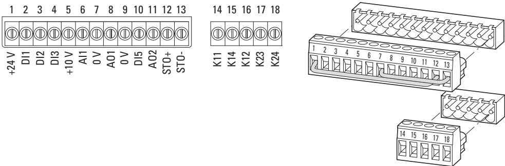
Abbildung 76: Benennung der steckbaren Steuerklemmen
