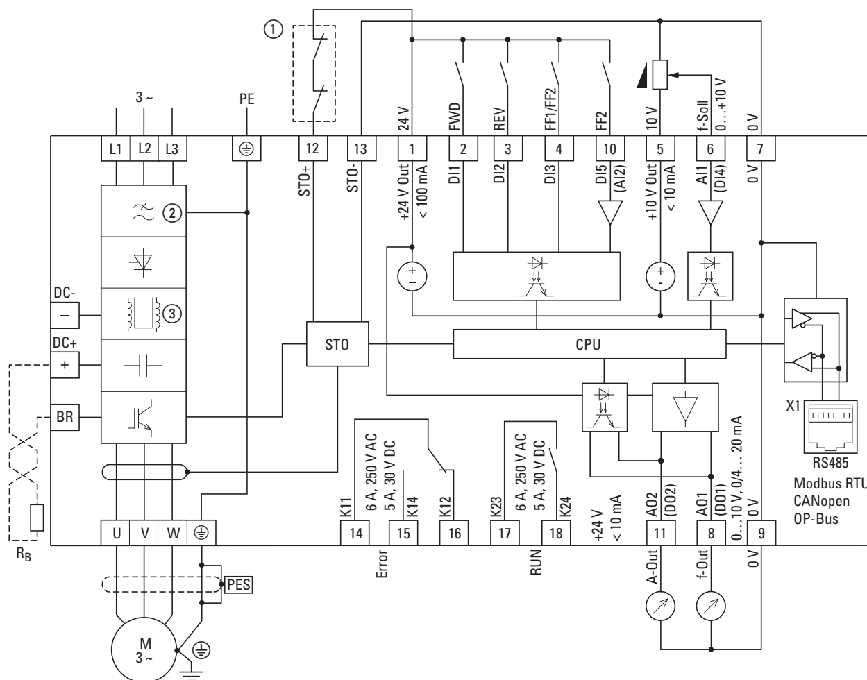
Abbildung 87: Blockschaltbild DA1-...-B55C
