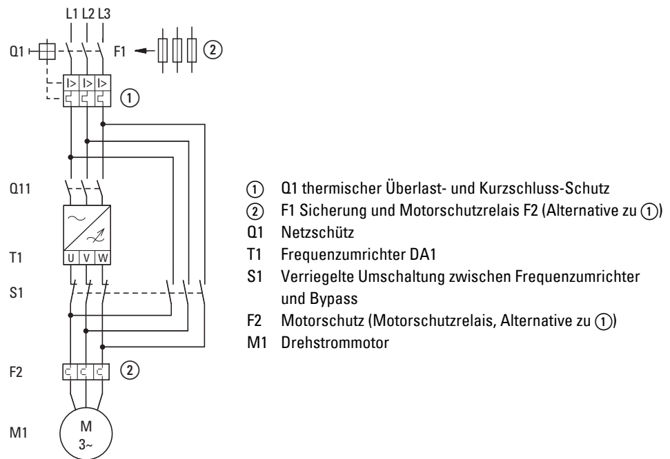
Abbildung 30: Bypass-Motorsteuerung (Beispiel)
