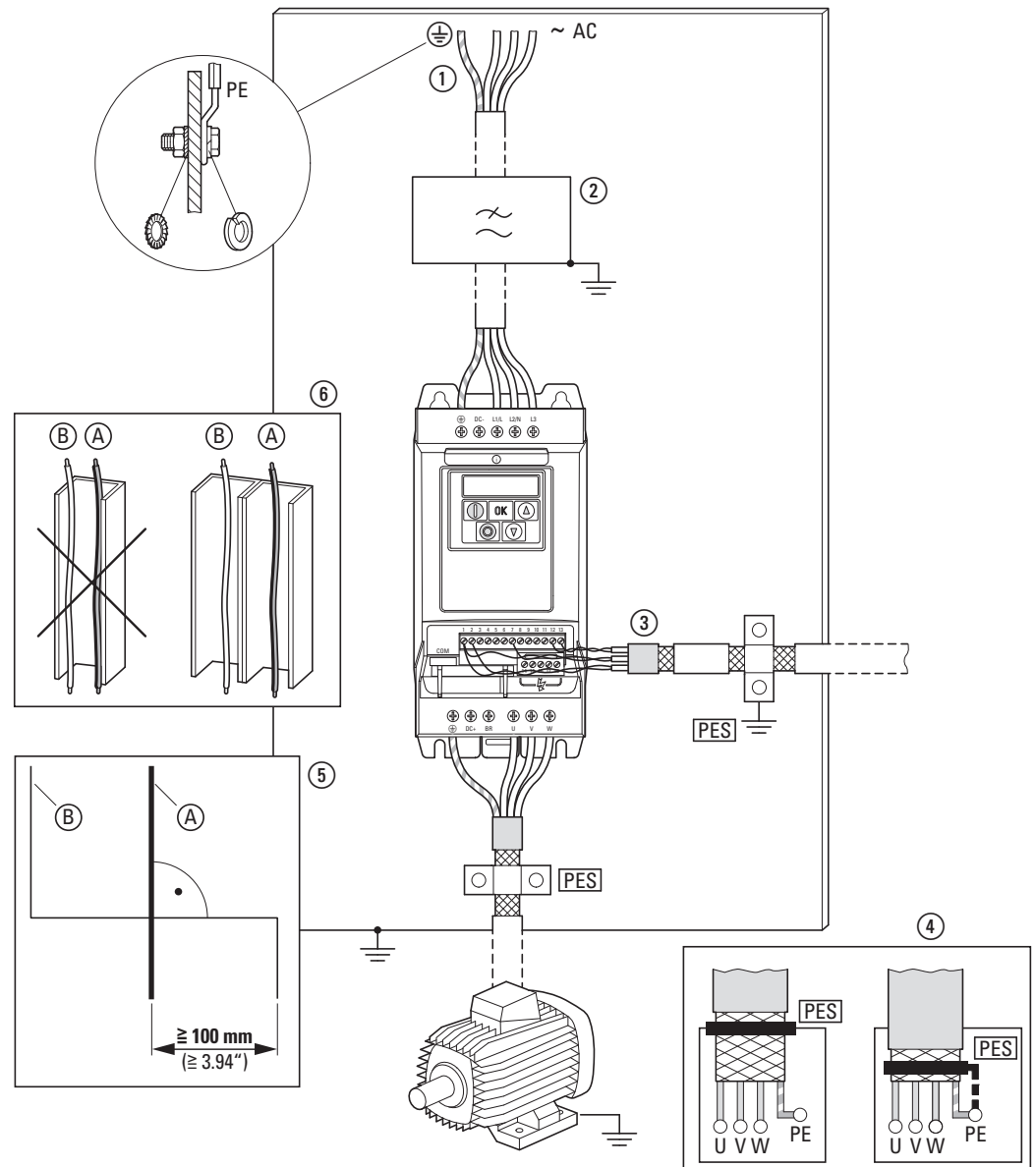
Abbildung 58: EMV-gerechte Installation
