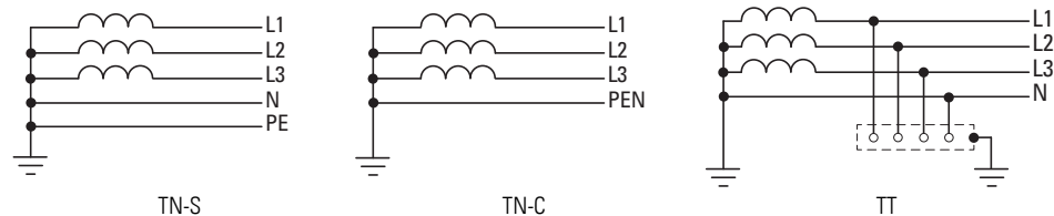
Abbildung 29: Wechselstromnetze mit geerdetem Mittelpunkt
