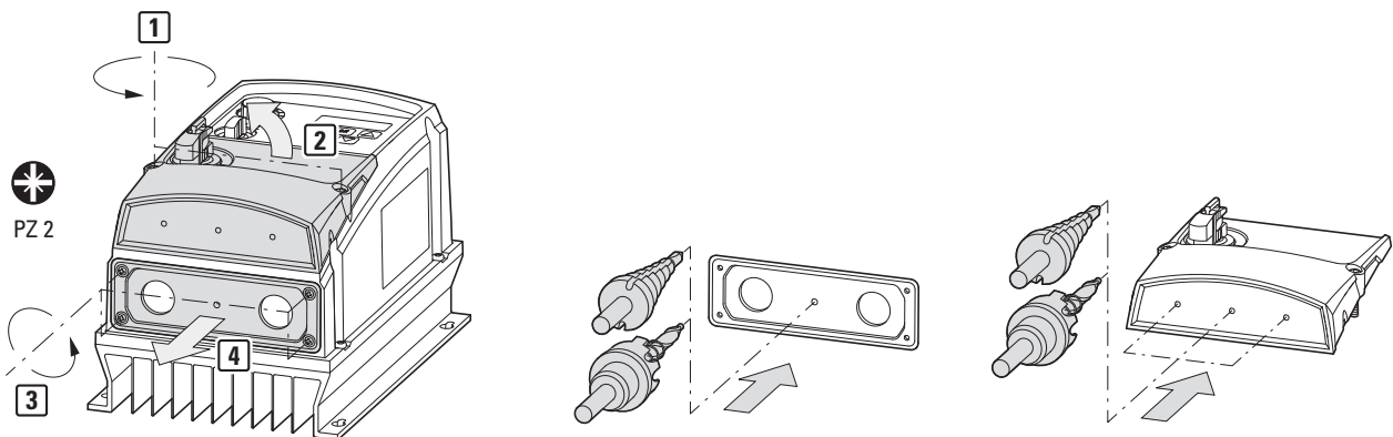
Abbildung 73: Bohrungen
