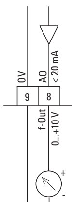
Abbildung 81: Analogausgang (AO) (Anschlussbeispiel)
