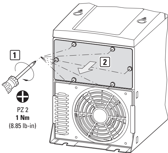
Abbildung 62: Abdeckplatte entfernen
