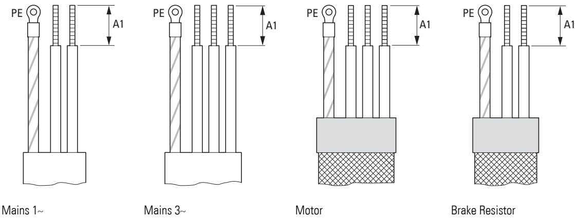
Abbildung 67: Anschlussleitungen
