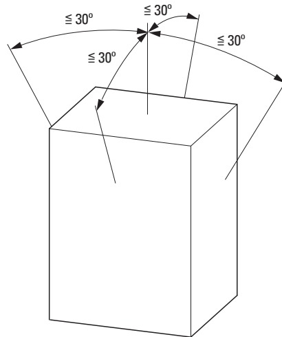
Abbildung 41: Einbaulage
