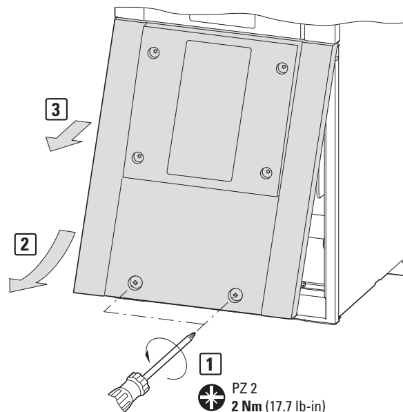
Abbildung 61: Deckel entfernen
