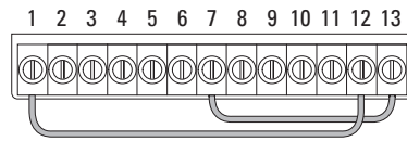
Abbildung 77: STO-Steuerklemmen (direkte Freigabe)
