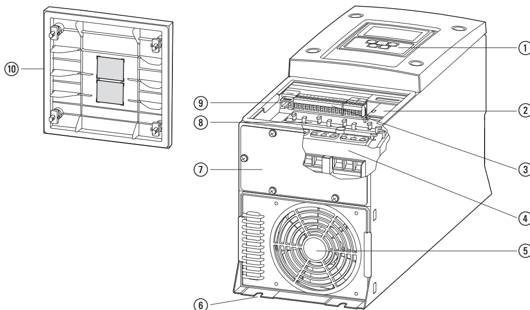
Abbildung 9: Benennungen am DA1 (hier: FS4, IP55)
