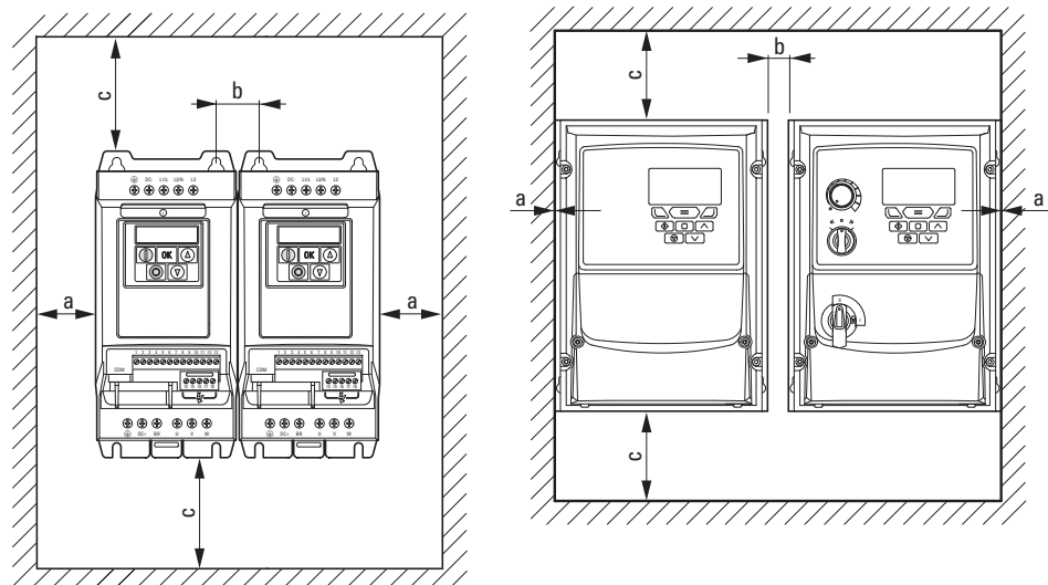
Abbildung 42: Freiräume zur Luftkühlung (links: IP20, rechts: IP66)
