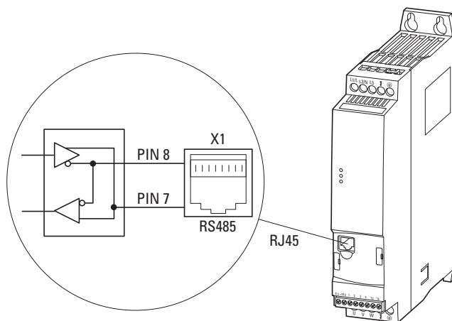
Figura 43: Interfața RJ45
