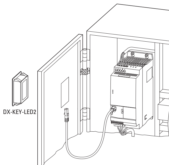
Figura 75: Montarea pe ușa dulapului de comandă
