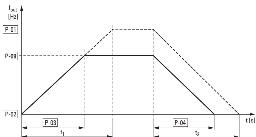
Figura 62: Timpul de accelerare și timpul de decelerare
