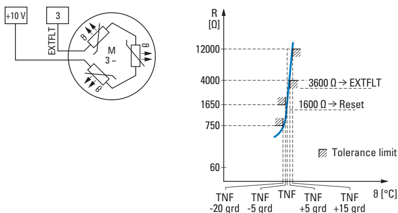
Figura 65: Exemplu de conectare a unui termistor și caracteristică de declanșare
