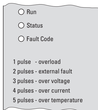
Figura 45: LED-urile cu codurile erorilor (imprimare pe carcasă)
