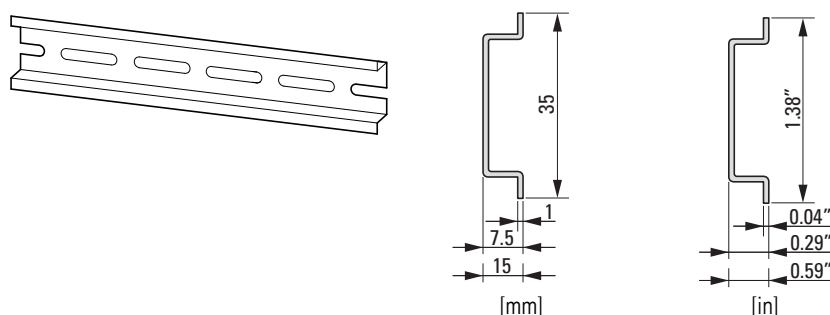
Figura 26: Șină de montaj conformă cu norma CEI/EN 60715
