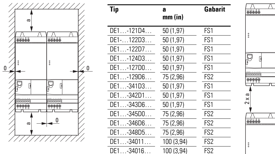
Figura 23: Spații libere pentru răcirea cu aer
