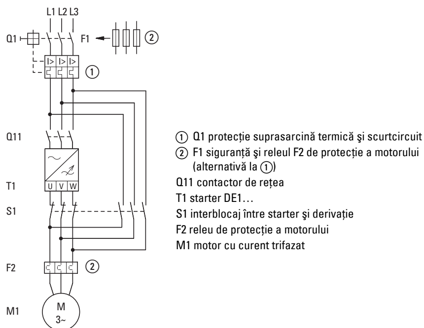
Figura 16: Schema de comandă cu bypass a motorului (exemplu)
