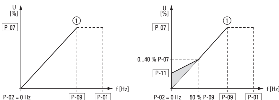
Figura 66: Caracteristica U/f
