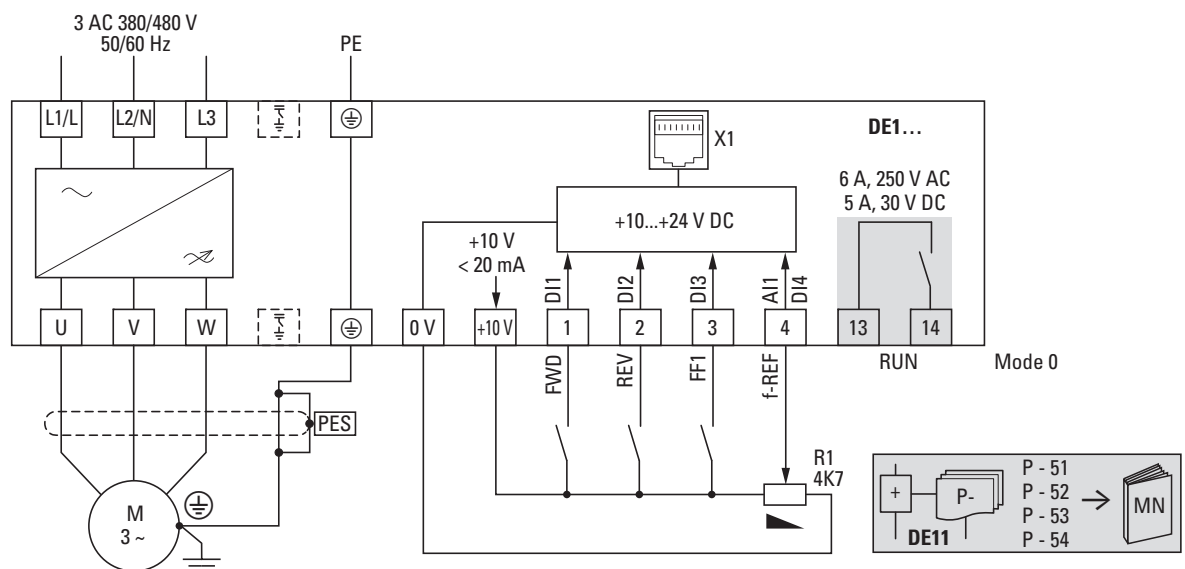
Figura 49: Schema bloc DE1-34...NN-... Starter cu tensiune trifazică de alimentare de la rețea și fără filtru intern de interferență radio
