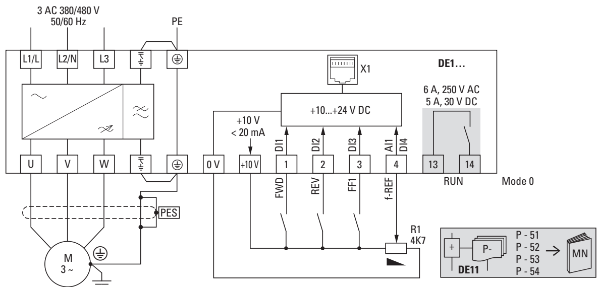
Figura 48: Schema bloc DE1-34...FN... Starter cu tensiune trifazică de alimentare de la rețea și filtru intern de interferență radio
