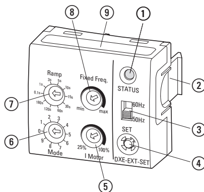
Figura 51: Componentele modulului DXE-EXT-SET
