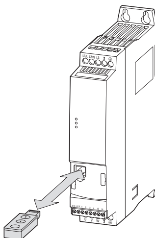
Figura 77: DE1... e DX-COM-STICK3
