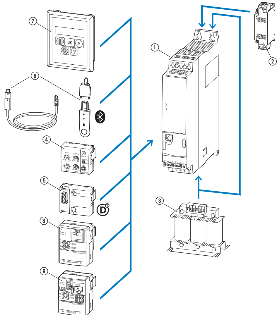
Figura 2: Composizione del sistema (Esempio)
