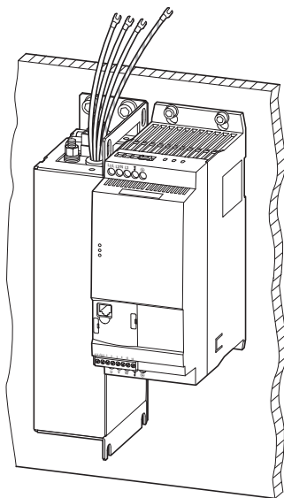
Figura 85: Disposizione di montaggio (esempio: DX-EMC34-019... e DE1...-340... nella grandezza FS2)
