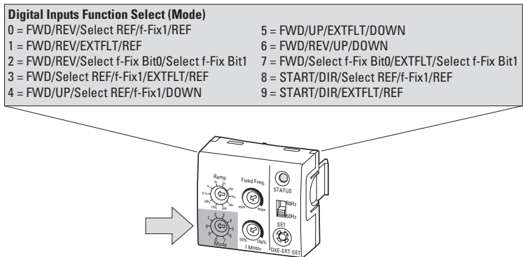
Figura 69: Modulo di configurazione DXE-EXT-SET
