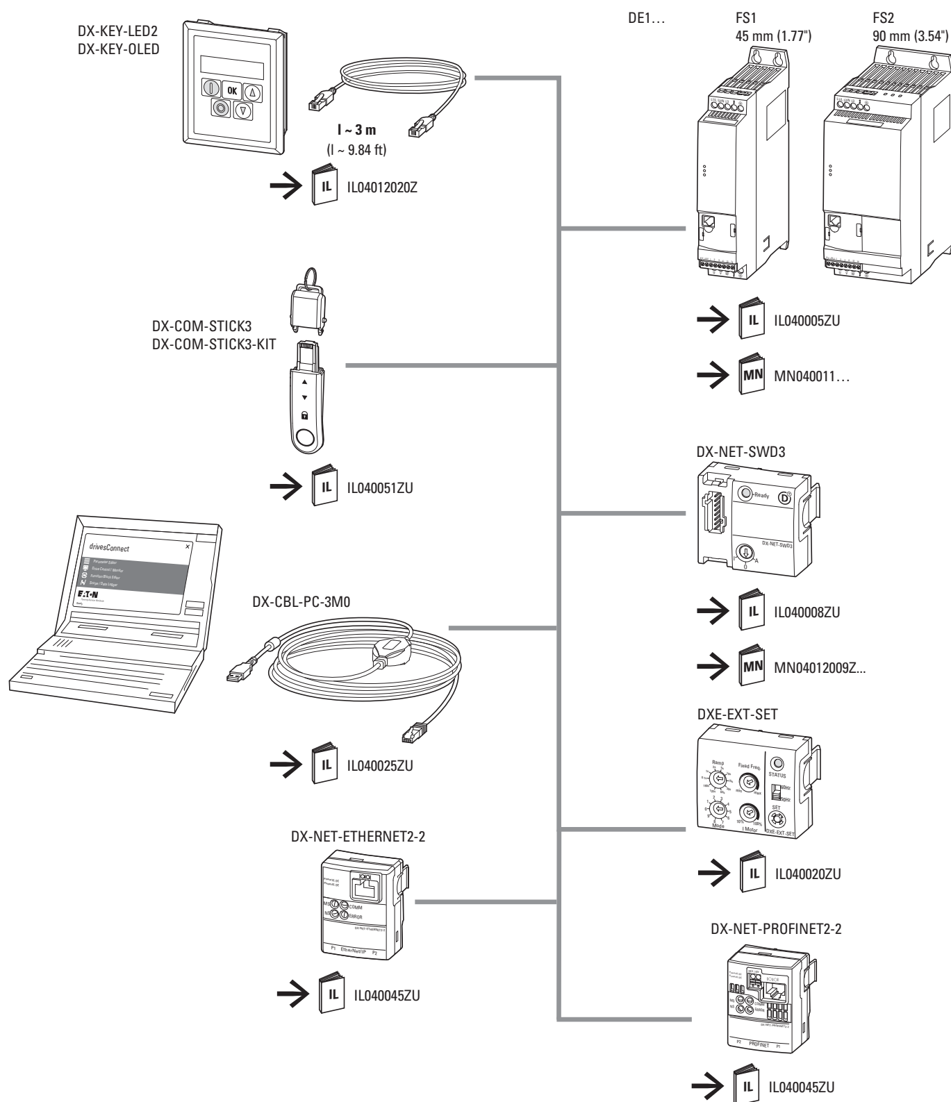
Figura 44: Composizione del sistema dell'interfaccia RJ45 dell'avviatore a velocità variabile DE1
