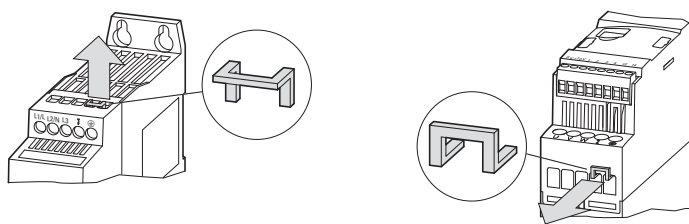
Figura 34: Rimozione dei ponticelli di collegamento EMC sul lato rete e sul lato motore
