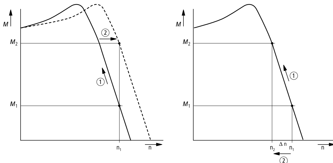
Figura 67: Comportamento in velocità con e senza compensazione dello scorrimento.
