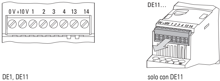
Figura 38: Disposizione dei morsetti di collegamento sulla porta di comando
