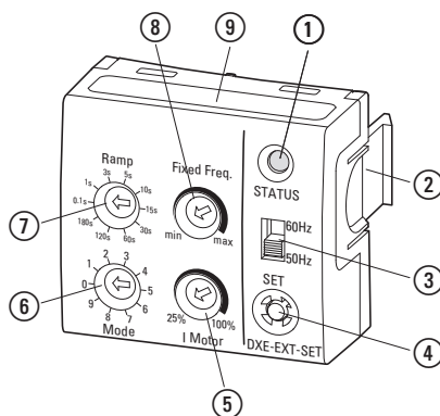
Figura 51: Designazioni su DXE-EXT-SET
