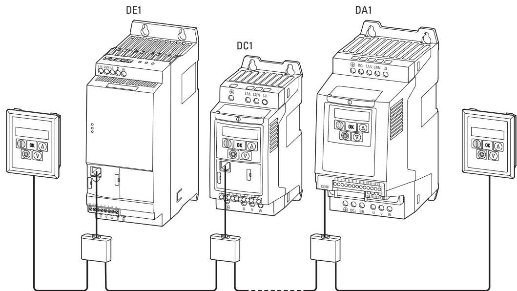
Figura 76: Esempio: rete PowerXL (OP-Bus) con due organi di comando
