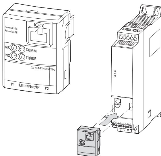
Figura 60: DX-NET-ETHERNET2-2 Modulo Ethernet/IP
