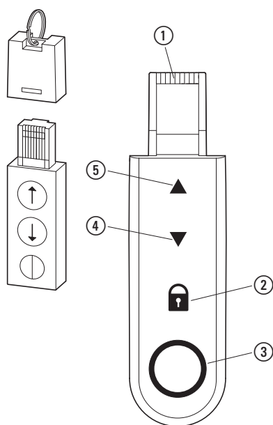
Figura 77: DE1... e DX-COM-STICK3
