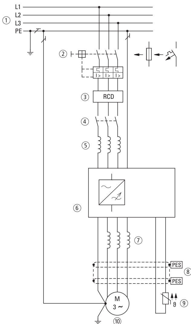
Figura 14: Esempio di sistema di azionamento con alimentazione trifase per un motore a corrente trifase
