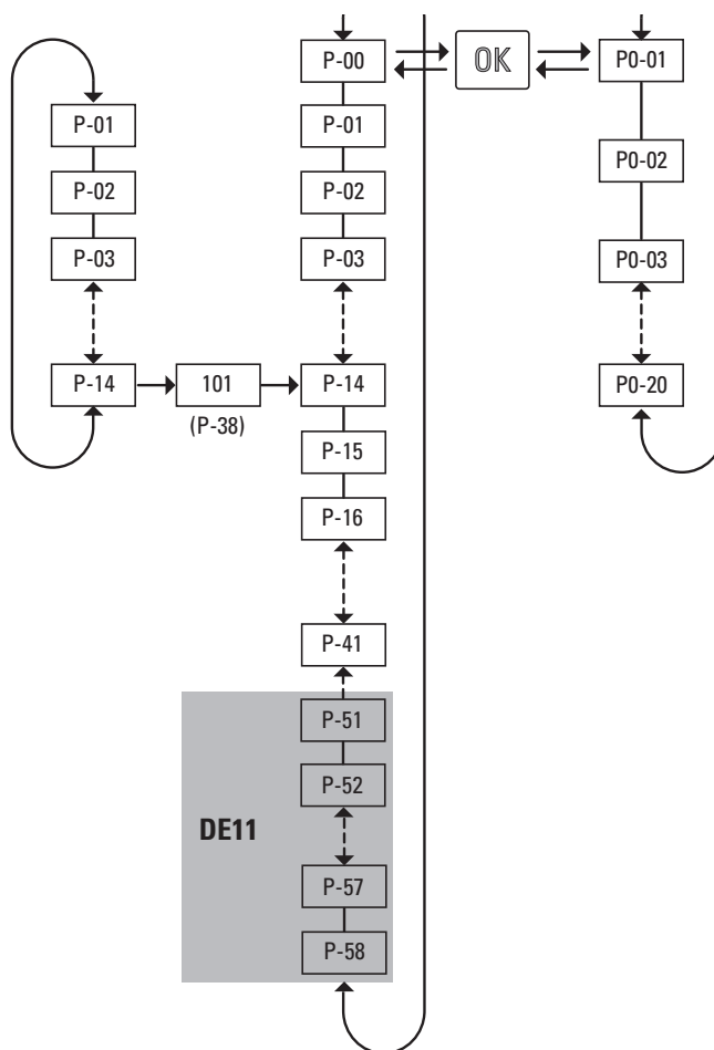
Figura 57: Struttura dei parametri
