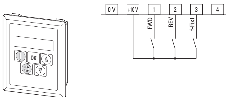
Figura 70: Organo di comando opzionale DX-KEY-LED2 e morsetto di comando P-15 = 0 (impostazione di fabbrica, modalità 0)
