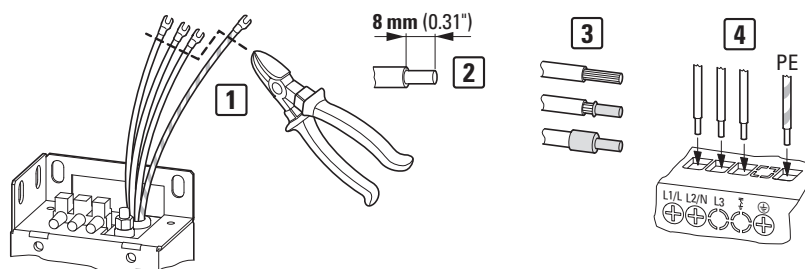
Figura 86: Adattamento dei cavi di collegamento preconfezionati
