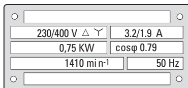
Figura 19: Esempio di targa dati (targhetta dati macchina) di un motore
