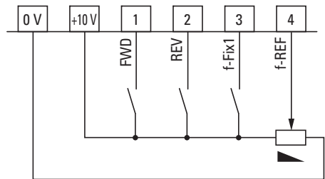
Figura 68: Impostazione di fabbrica dei morsetti di comando
