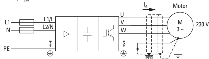
Figura 10: DE1...-12...NN-N20N (senza filtro soppressione radiodisturbi)
