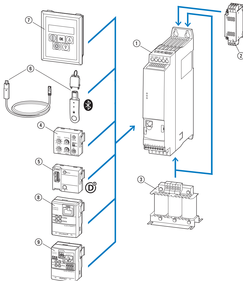
Figura 2: Sinóptico del sistema (ejemplo)
