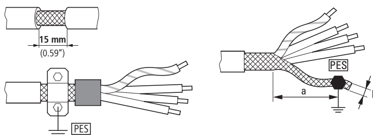
Figura 36: Cable de conexión apantallado en el circuito del motor
