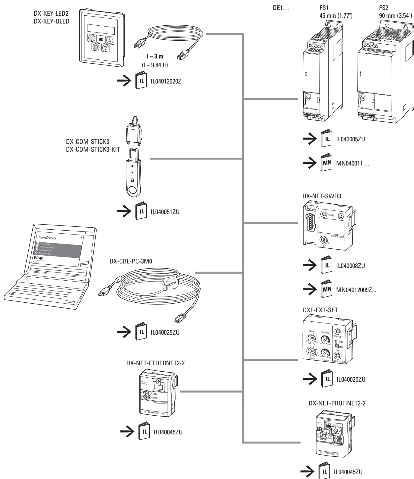
Figura 44: Sinóptico del sistema para la interfaz RJ45 del arrancador de velocidad variable DE1
