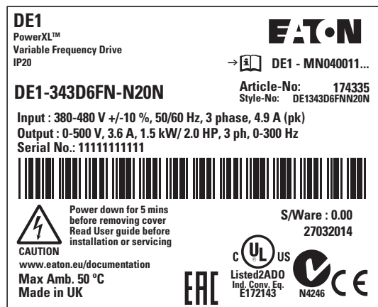
Figura 5: Etiqueta de características A (colocada lateralmente)
