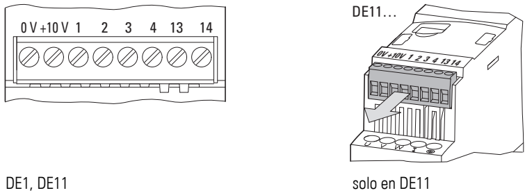
Figura 38: Disposición de los bornes de conexión en el circuito de control
