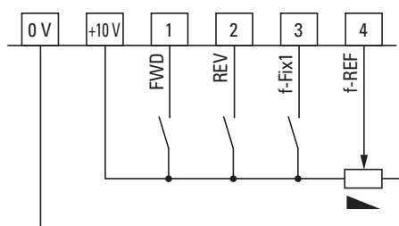
Figura 68: Configuración de serie de los terminales de control
