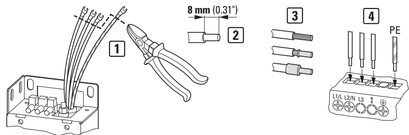
Figura 86: Adaptación de los cables de conexión confeccionados.
