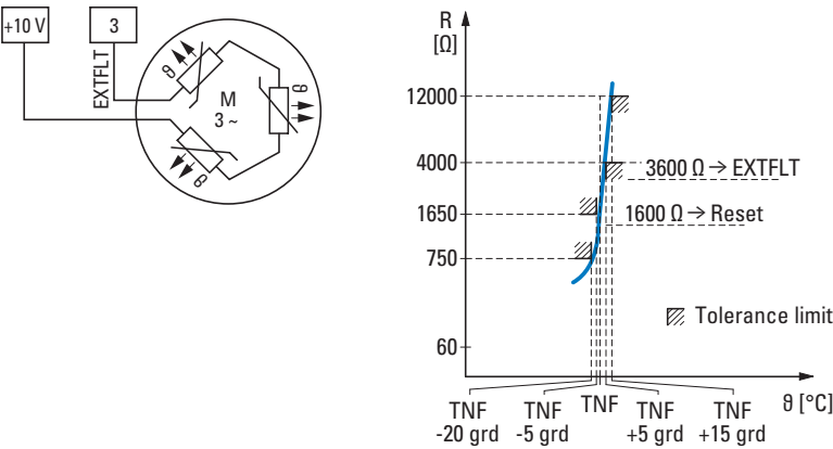
Figura 65: Ejemplo de conexión termistor y curva característica de disparo
