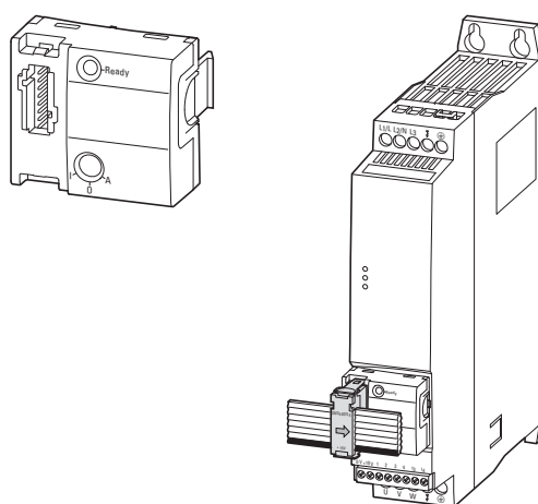
Figura 59: Módulo de conexión SWD DX-NET-SWD3
