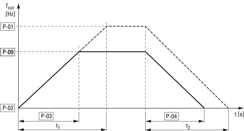
Figura 62: Tiempo de aceleración y deceleración
