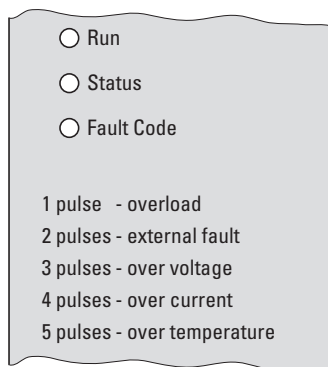
Figura 45: Indicaciones LED con códigos de error (impresión en el envoltente)
