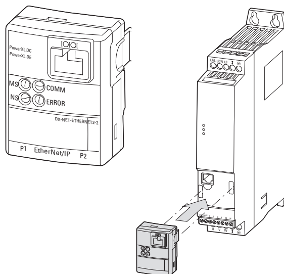
Figura 60: DX-NET-ETHERNET2-2 Módulo EtherNet/IP
