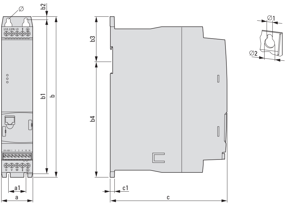
Figura 73: Dimensiones
