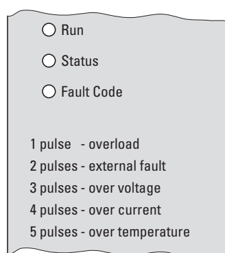
Figura 88: Indicaciones LED con mensaje de error
