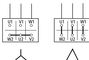
Figura 64: Tipos de conexiones (triángulo, estrella)
