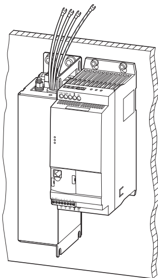
Figura 85: Disposición de montaje (ejemplo: DX-EMC34-019... y DE1...-340... en el tamaño FS2)
