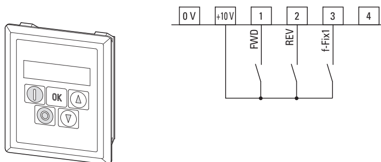
Figura 70: Unidad de mando opcional DX-KEY-LED2 y terminal de control P-15 = 0 (configuración de serie, modo 0)
