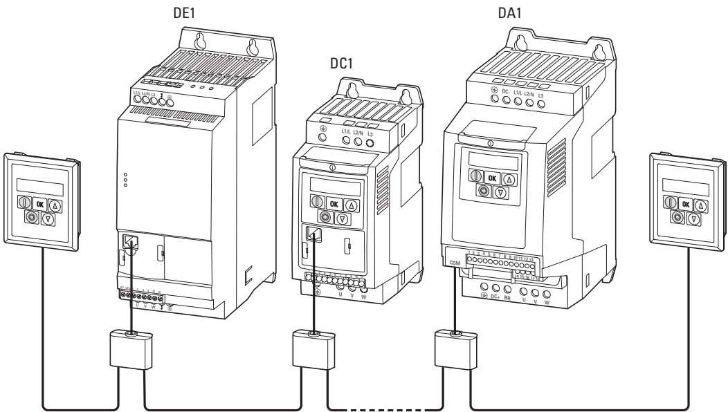
Figura 76: Ejemplo: red PowerXL (bus PO) con dos unidades de mando
