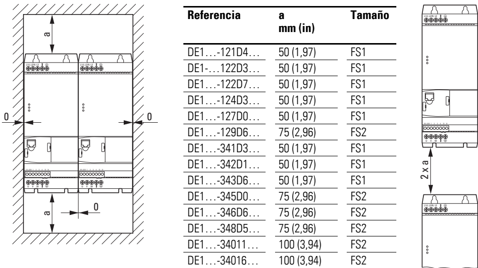
Figura 23: Espacios libres para la refrigeración de aire
