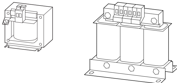
Figura 83: Reactancias de red DEX-LN...
