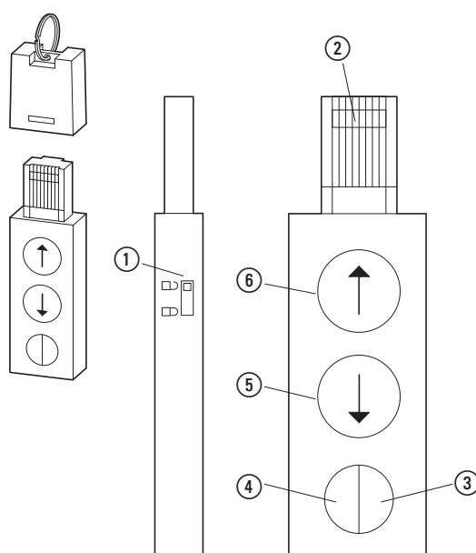
Figura 78: DX-COM-STICK3
