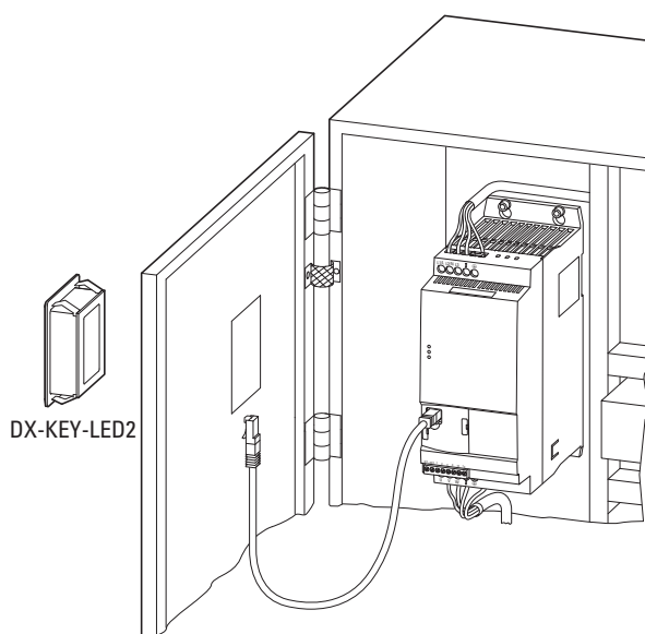
Figura 75: Montaje en una puerta del armario eléctrico
