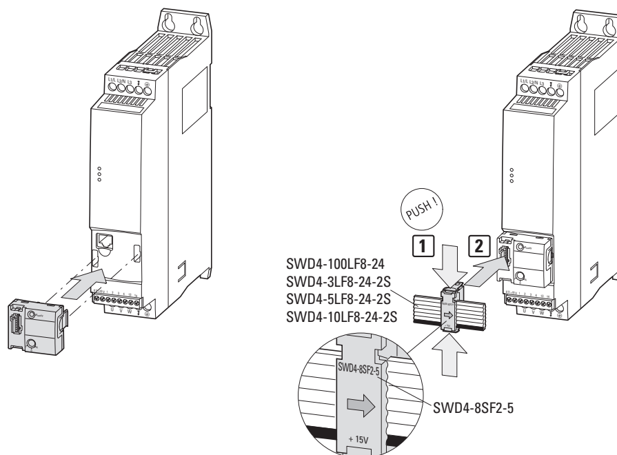
Figura 80: Conexión SmartWire-DT
