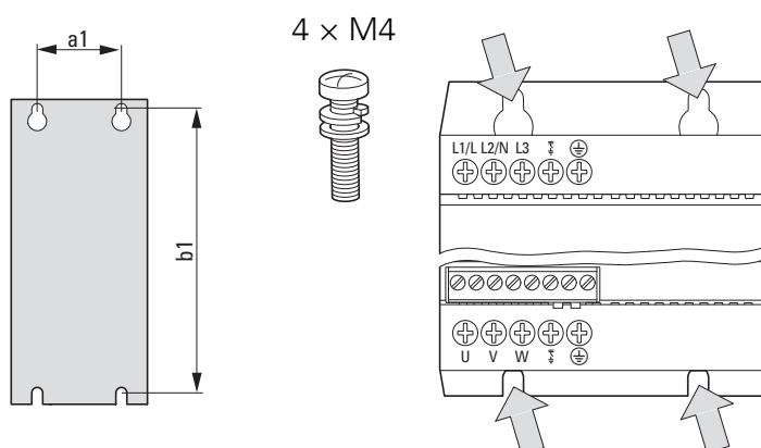
Figura 25: Fijación por tornillo
