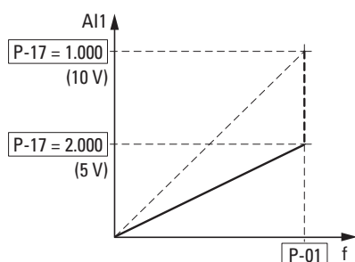
Figura 71: Entrada de valores de consigna escalada
