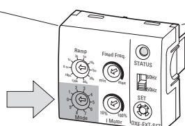
Figura 69: Módulo de configuración DXE-EXT-SET
