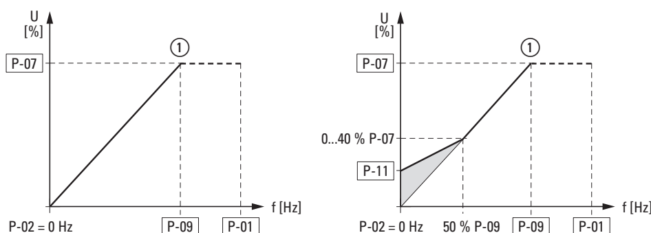
Figura 66: Curva característica U/f
