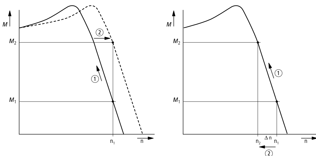
Figura 67: Comportamiento de velocidad con y sin compensación de deslizamiento.
