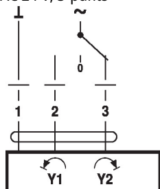
Aansluitschema's AC 24 V, 3-punts
