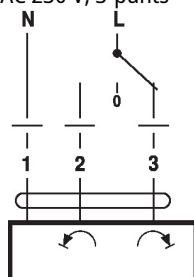
Aansluitschema's AC 230 V, 3-punts
