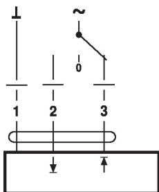
Aansluitschema's AC 24 V, 3-punts
