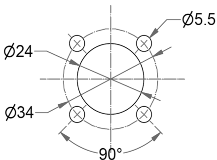
Bohrbild LC D3-2 von 160-315A
