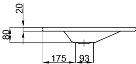
Abb.: BetteAqua 1400 x 495 mm mit 2 Hahnlöchern
