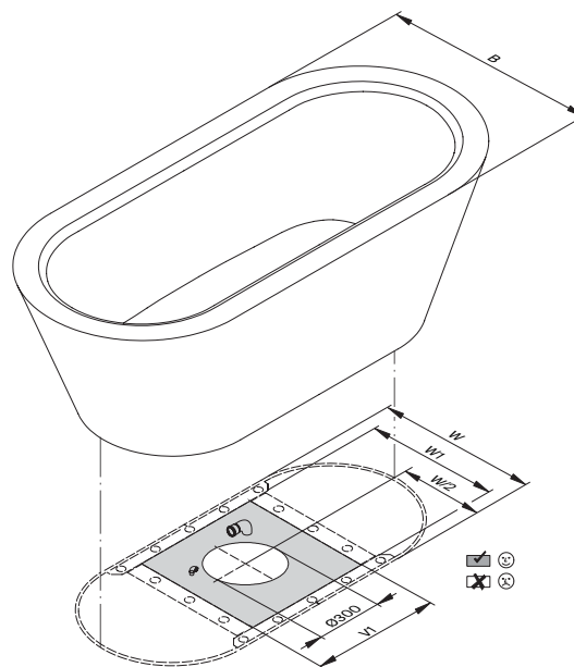
Aansluitmaat voor af- en overlopgarnituur
