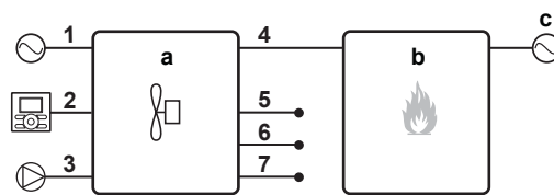
a Buitenunit b Gasboiler van derden c Elektrische voeding voor gasboiler
