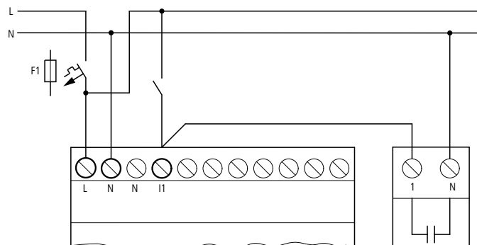
Abbildung 17: easy mit EASY256-HCI
