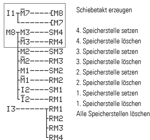
Abbildung 86: easy-Schaltplan Schieberegister
