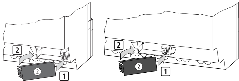
Abbildung 99: Speicherkarte stecken
