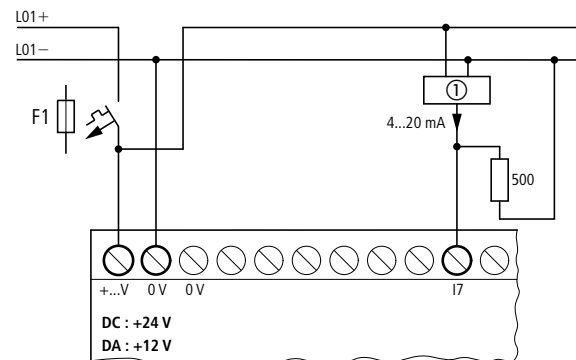
Abbildung 25: Anschluss 0 (4) bis 20 mA Sensorausgang, Analog-Eingang
