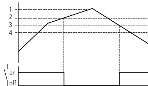
Abbildung 49: Wirkdiagramm Analogwertvergleich Betriebsart „kleiner als“
