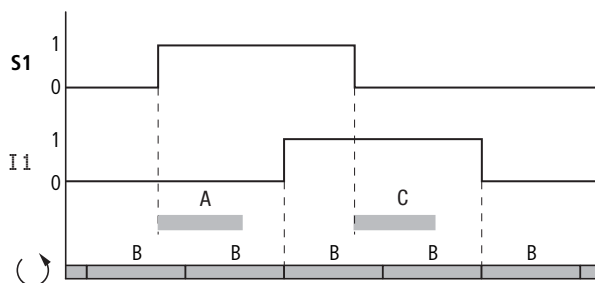
Abbildung 92: Verzögerungszeiten von easy-DC und easy-DA
