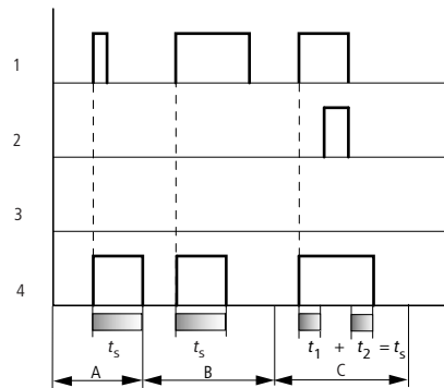
Abbildung 70: Wirkiagramm Zeitrelais, Impulsformend 1
