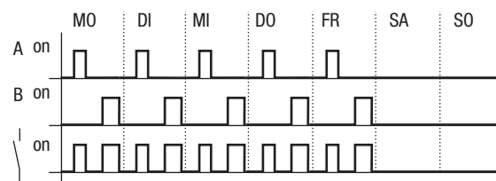
Abbildung 59: Wirkdiagramm „Arbeitstage“
