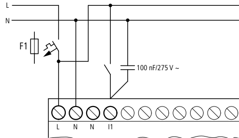
Abbildung 15: Erhöhung des Eingangsstromes
