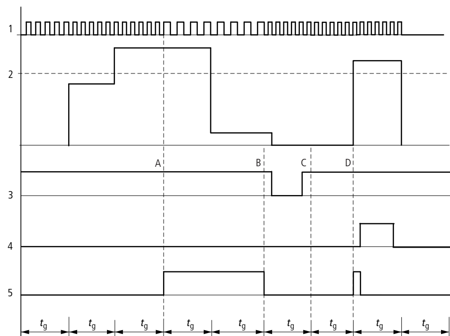
Abbildung 56: Wirkdiagramm Frequenzzähler
