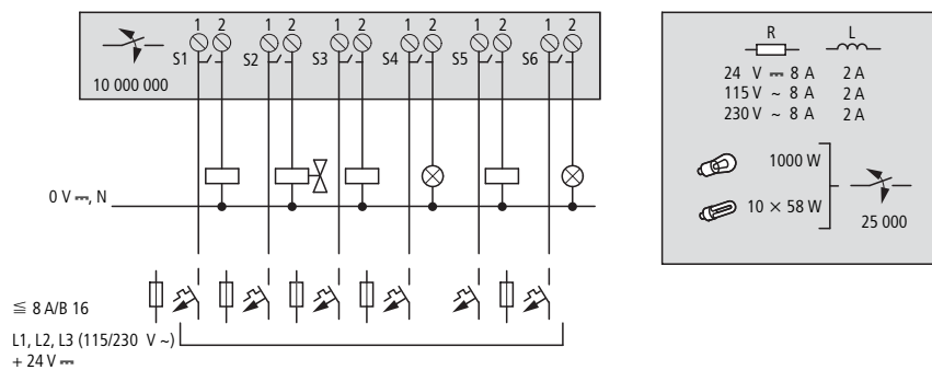
Abbildung 30:Relais-Ausgänge EASY618...-RE
