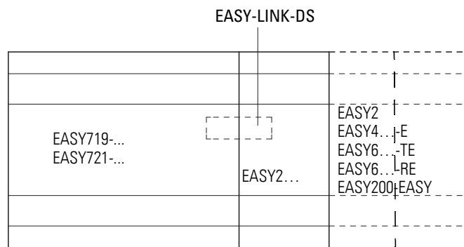
Abbildung 35: Lokale Erweiterung mit dem Basisgerät verbinden
