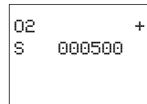
Parametereinstellung des Zeitrelais T1
