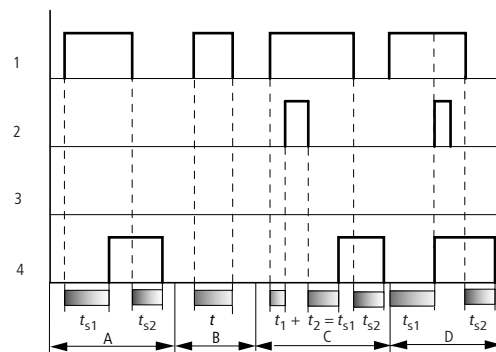
Abbildung 67: Wirkdiagramm Zeitrelais, ansprech- und rückfallverzögert 1
