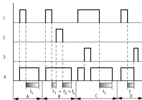
Abbildung 65: Wirkdiagramm Zeitrelais rückfallverzögert (mit/ohne Zufallsschalten)
