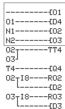
Schaltplandarstellung
