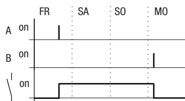
Abbildung 60:Wirkdiagramm „Wochenende“
