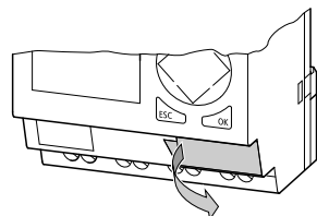
Abbildung 98: Schnittstellenabdeckung entfernen
