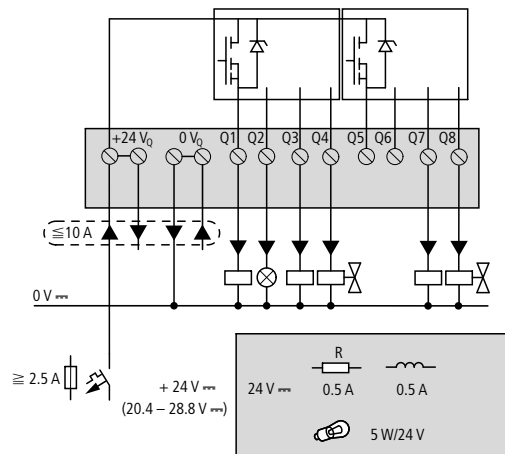
Abbildung 32: Transistor-Ausgänge EASY7...-T..
