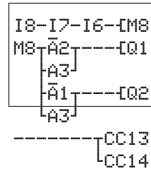
Schaltplandarstellung
