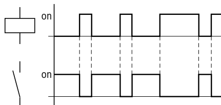
Abbildung 41: Wirkdiagramm inverse Schützfunktion
