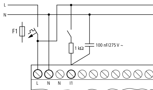
Abbildung 16: Begrenzung des Eingangsstromes durch Widerstand
