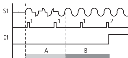
Abbildung 95: Taster, der prellt
