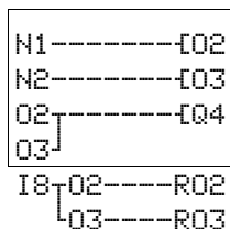
Schaltplandarstellung
