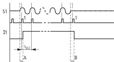
Abbildung 94: Einschaltverzögerung easy-AC und easy-AB
