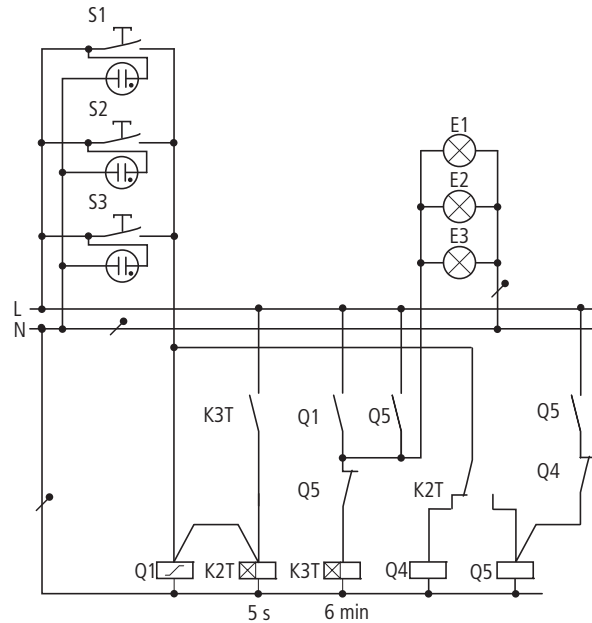
Abbildung 88: Konventionelle Treppenhausbeleuchtung
