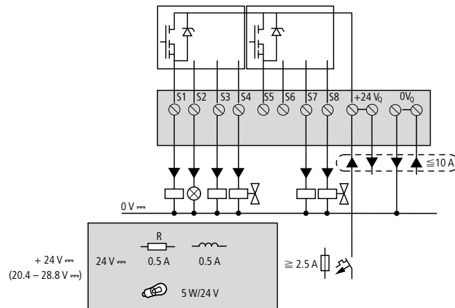
Abbildung 33: Transistor-Ausgänge EASY620-..-TE
