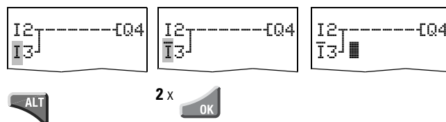
Abbildung 39: Kontakt I3 von Schließer zu Öffner ändern
