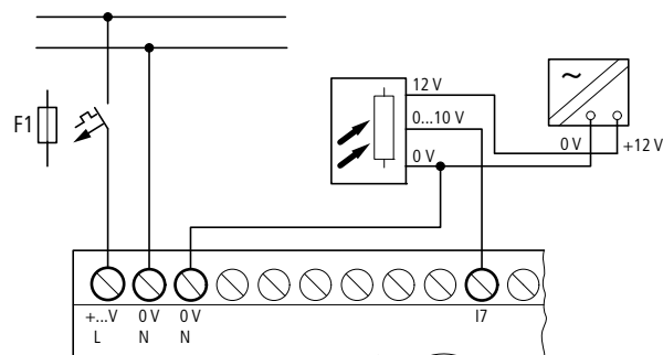
Abbildung 23:Anschluss eines Helligkeitssensors, Analog-Eingang
