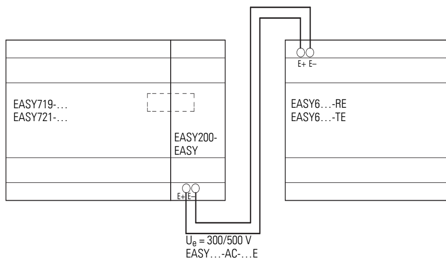
Abbildung 36: Dezentrale Erweiterung an easy anschließen
