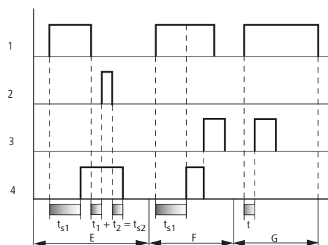
Abbildung 68: Wirkdiagramm Zeitrelais, ansprech- und rückfallverzögert 2
