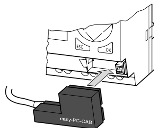
Abbildung 100: Programmierleitung stecken
