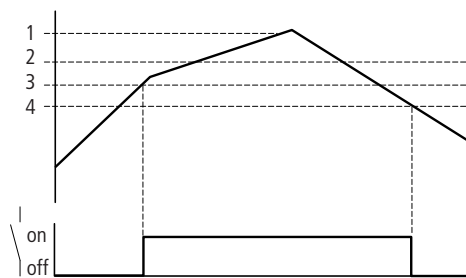
Abbildung 52:Wirkdiagramm Analogwertvergleich Betriebsart „größer gleich“
