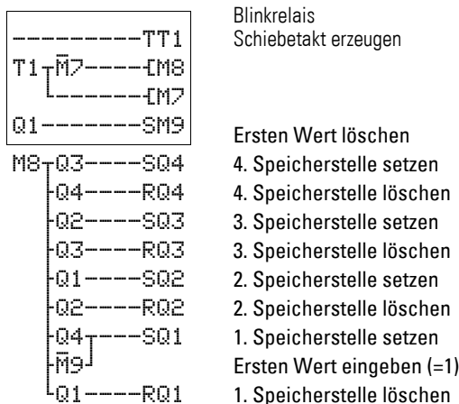
Abbildung 87: easy-Schaltplan Lauflicht
