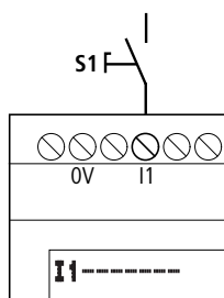
Abbildung 91: easy-Eingang mit Schalter belegt
