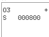
Parametereinstellungen des Betriebsstundenzählers 03
