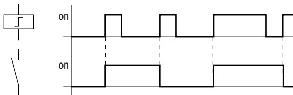
Abbildung 44: Wirkdiagramm Stromstoßrelais
