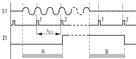
Abbildung 96: Ein- und Ausschaltverhalten
