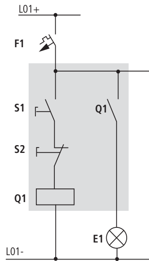
Abbildung 37: Lampensteuerung mittels Relais
