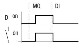
Abbildung 61:Wirkdiagramm „Nachtschalten“
