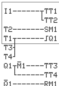
Abbildung 90: easy-Schaltplan Treppenhaus
