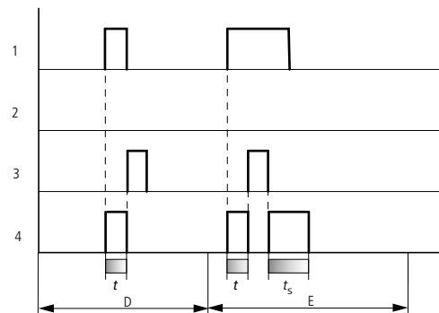
Abbildung 71: Wirkiagramm Zeitrelais, Impulsformend 2
