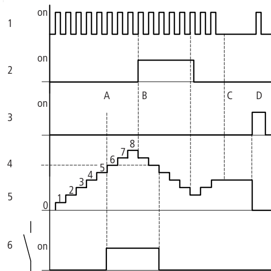
Abbildung 54: Wirkdiagramm
