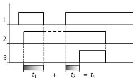
Abbildung 73: Wirkungweise der Schaltung
