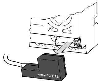
Abbildung 101:EASY-PC-CAB ziehen
