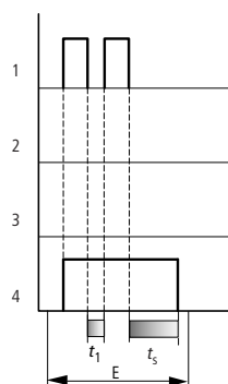
Abbildung 66: Wirkdiagramm Zeitrelais rückfallverzögert (mit/ohne Zufallsschalten, mit Retriggerung)
