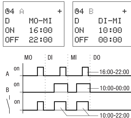
Abbildung 62: Wirkdiagramm „Zeitüberschneidungen“
