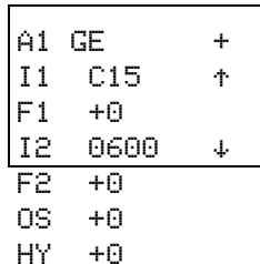
Parametereinstellungen des Analogwert-Vergleichers A1
