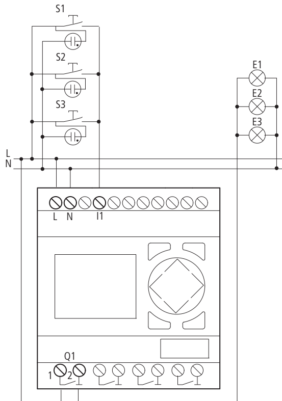
Abbildung 89: Treppenhausbeleuchtung mit easy
