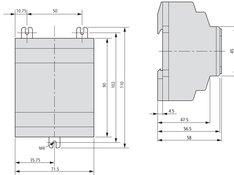
Abbildung 104: Abmessungen easy512-... in mm (Angaben in inches siehe Tabelle 36)
