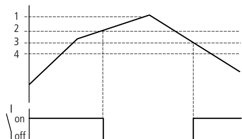
Abbildung 50: Wirkdiagramm Analogwertvergleich Betriebsart „kleiner gleich“
