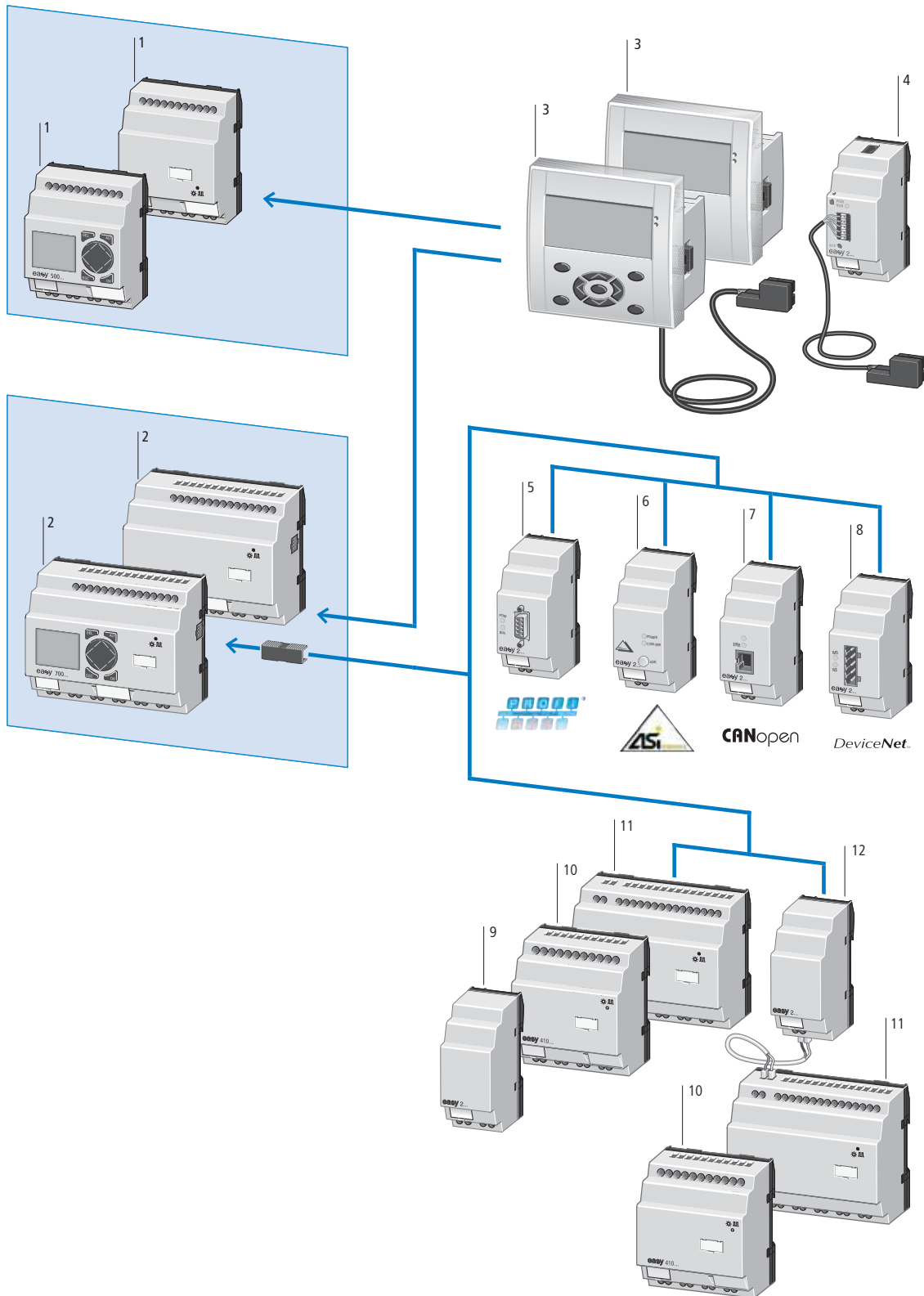
Abbildung 1: easy-Basisgeräte und -Erweiterungen
