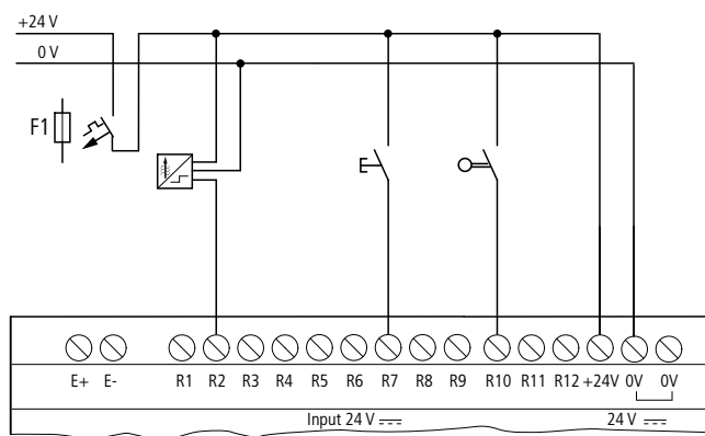
Abbildung 19: Digitale Eingänge anschließen EASY...-DC-.E
