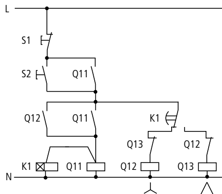
Abbildung 83: Stern-Dreieckschaltung mit herkömmlichen Schützen
