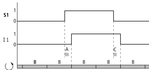
Abbildung 93: Schaltverhalten bei abgeschalteter Eingangsverzögerung
