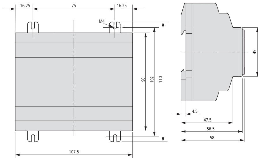
Abbildung 105: Abmessungen easy600, easy700 in mm (Angaben in inches siehe Tabelle 36)
