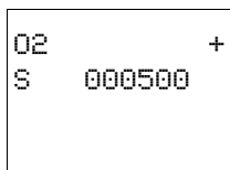
Parametereinstellungen des Betriebsstundenzählers 02
