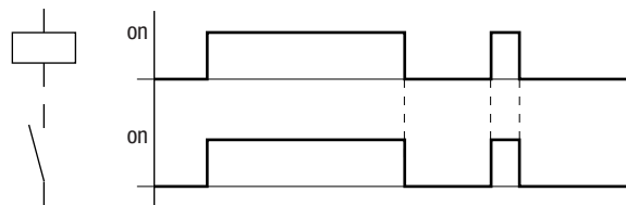
Abbildung 40: Wirkdiagramm Schützfunktion
