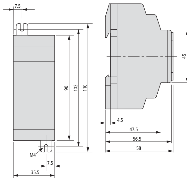
Abbildung 103: Abmessungen easy200 in mm (Angaben in inches siehe Tabelle 36, Seite 209)
