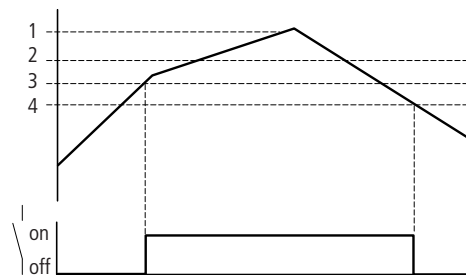
Abbildung 53: Wirkdiagramm Analogwertvergleich Betriebsart „größer als“
