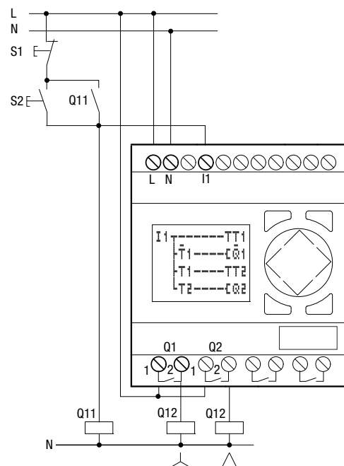
Abbildung 84: Stern-Dreieckschaltung mit easy
