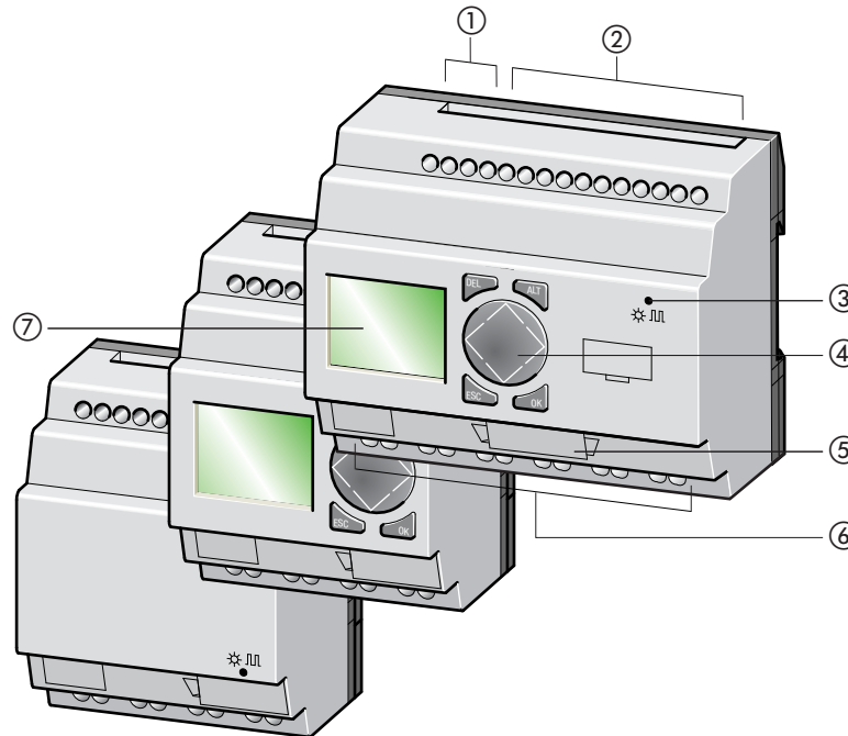
Abbildung 2: Geräteübersicht
