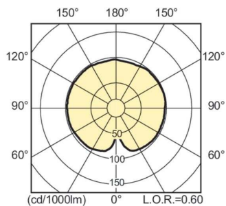
Light Distribution Diagram - MC CDM-Tm Elite Mini 20W/830 GU6.5 1CT
