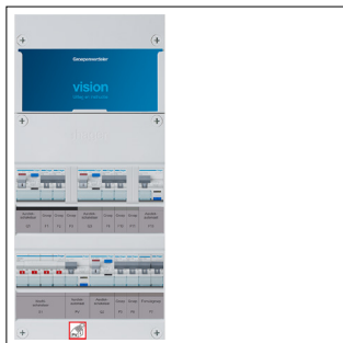
VKG222F63-AFR
