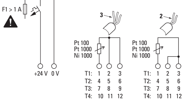
EASY-E4-DC-4PE1(P)
