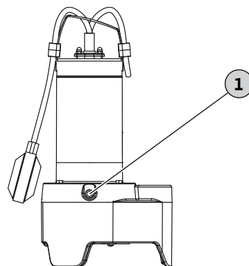
Fig. 3: Vidange d'huile de la chambre d'étanchéité
