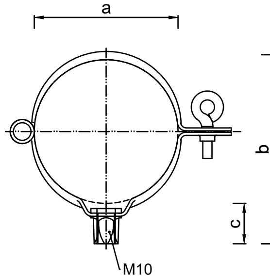
Bovenaanzicht
