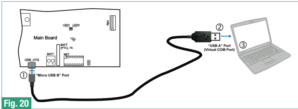
Fig. 20. Programmering met de LOGIPROG software
