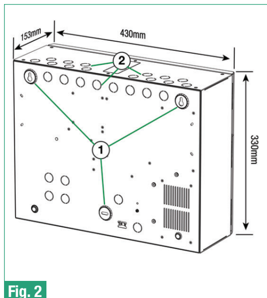
Fig. 2 – Montage-apparaten op de bodem:
