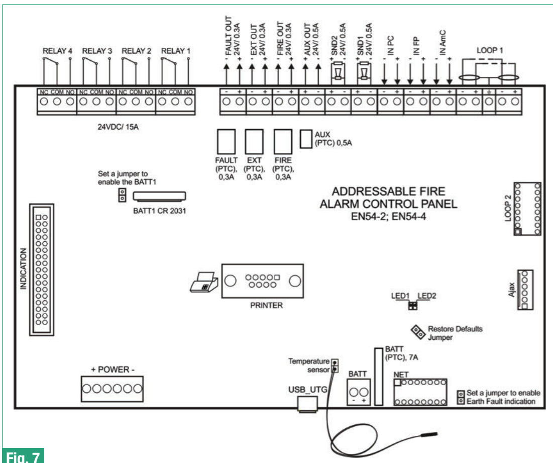
Fig. 7 – Moederbord van de brandmeldcentrale 41CPE112
