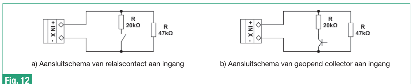
Fig. 12 – Aansluitvoorbeelden aan gespecialiseerde ingangen INXX
