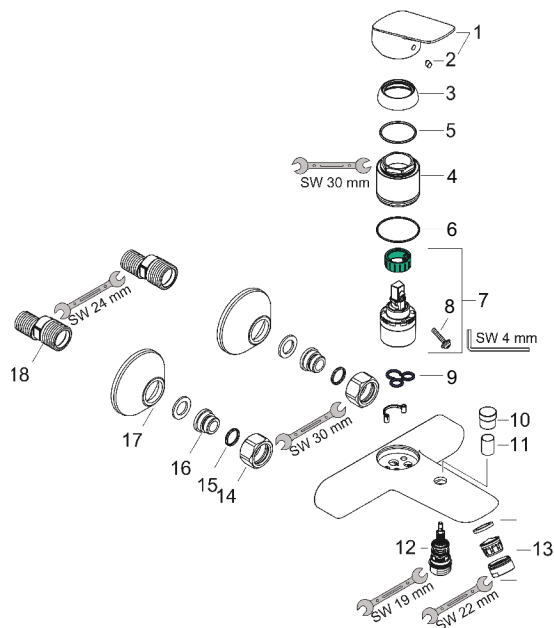
製品分解図
