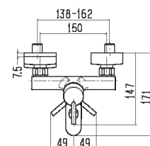
完成図
