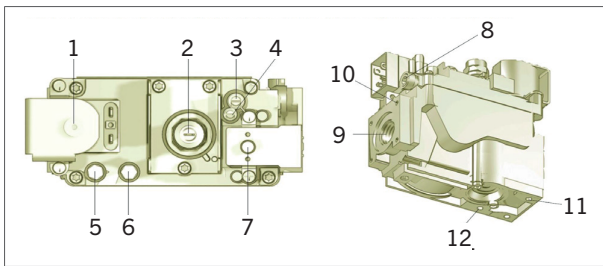
Abbildung 25 - Hauptkomponenten des Gasregelventils HR80 - 120
