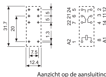
Aanzicht op de aansluitingen
