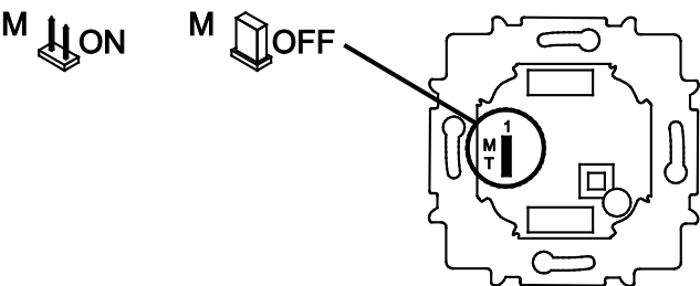
Afb. 3: 1511 U bewakingssokkel
