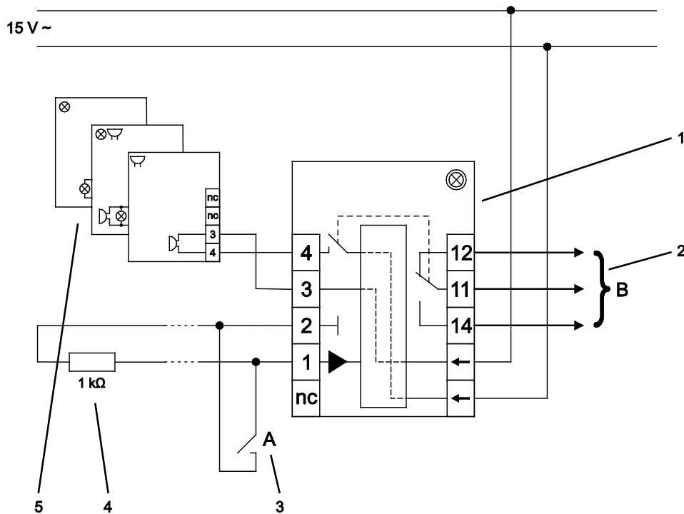
Afb. 1: Aansluitschema bewakingssokkel
