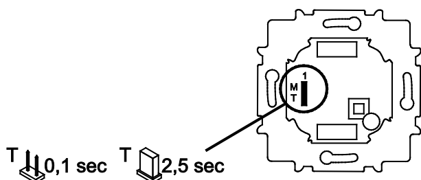
Afb. 4: 1511 U bewakingssokkel
