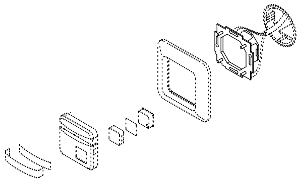
Afb. 2: Overzicht montage
