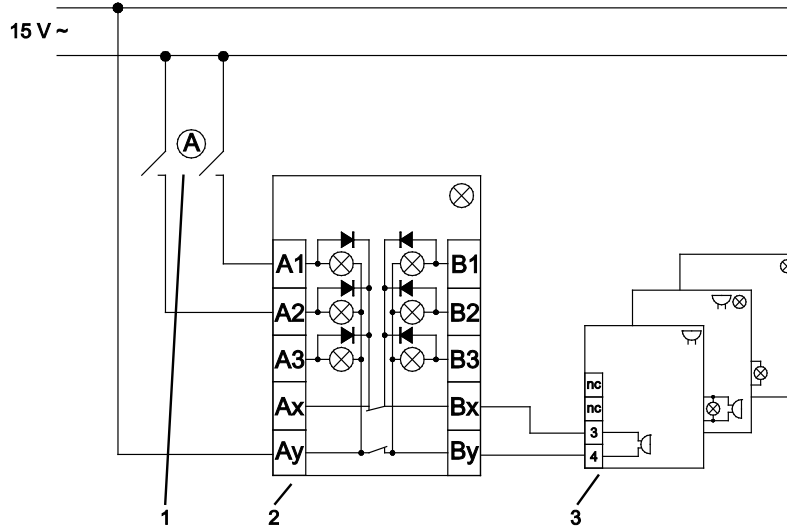
Abb. 1: Anschlussbild Alarmmelde-Einsatz als eine Gruppe
