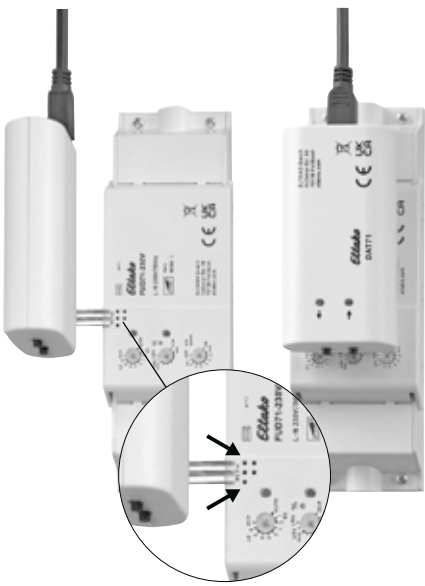
Aufstecken des Datenübertrager DAT71 auf einen Aktor der Baureihe 71.
