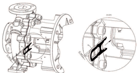
Fig. 47: 插入安装叉
