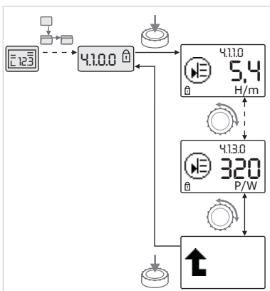
Fig. 46: 调用信息
