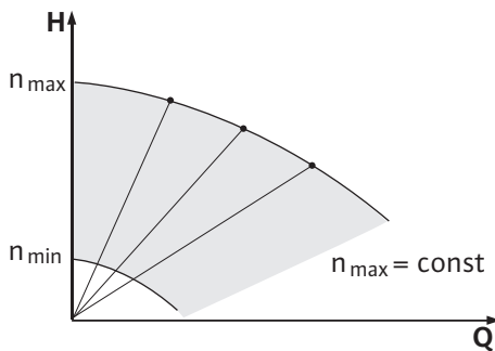
Fig. 33: 恒定转速
