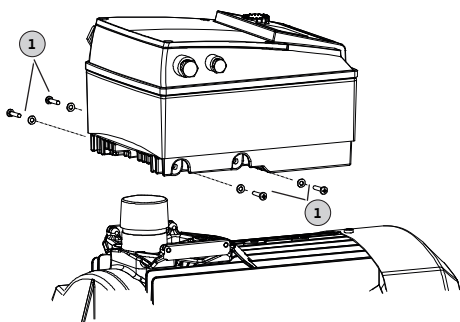
Fig. 48: 更换电气模块
