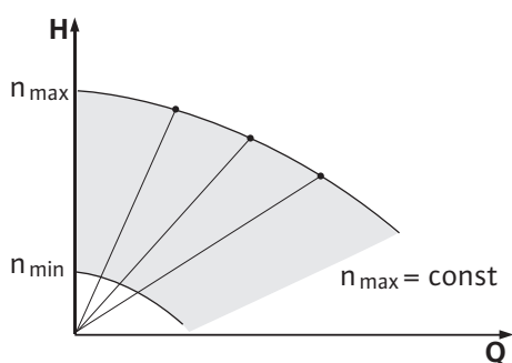
Fig. 8: 恒定转速
