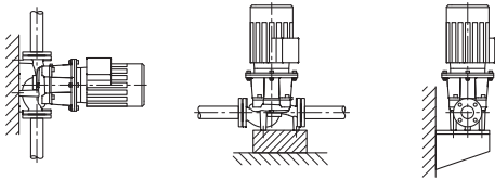
Fig. 3: IL-E视图
