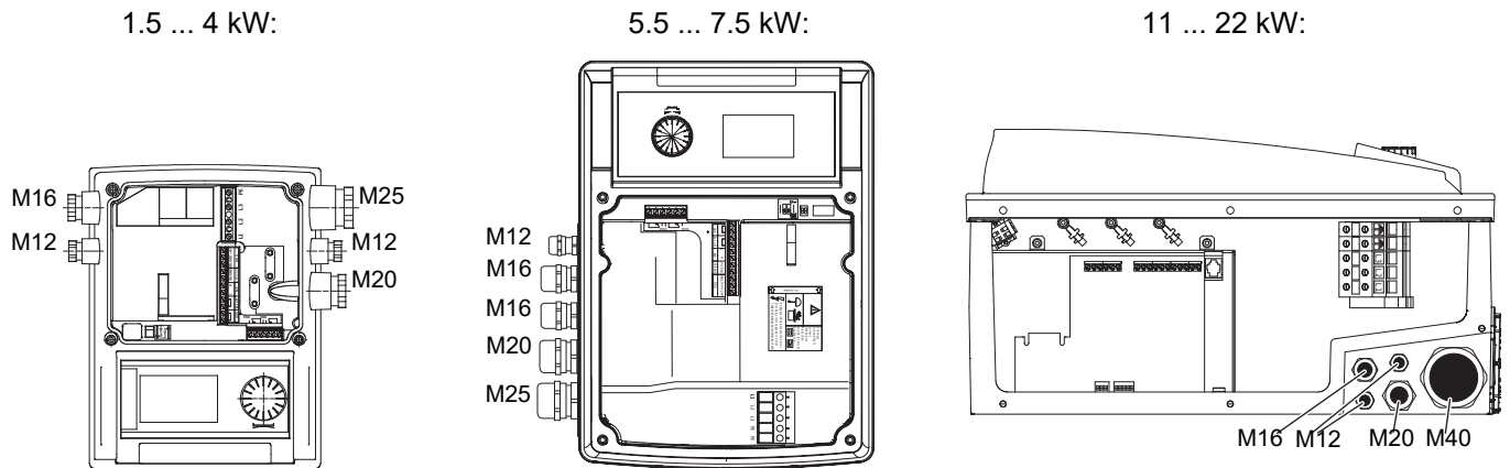
Fig. 29: 电缆螺纹连接
