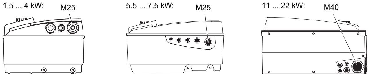
Fig. 24: 用于电源连接电缆的电缆螺纹接头
