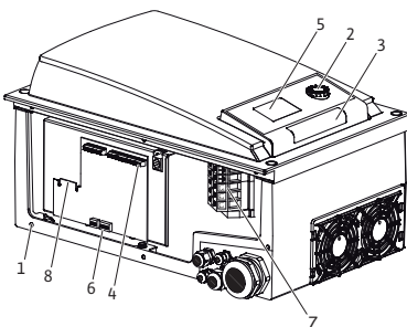
Fig. 5: 电子模块, 概览
