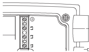
Fig. 27: 功率端子
