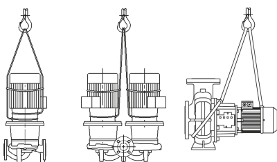
Fig. 1: 运输水泵
