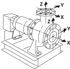
Fig. 22: 荷载条件1A
