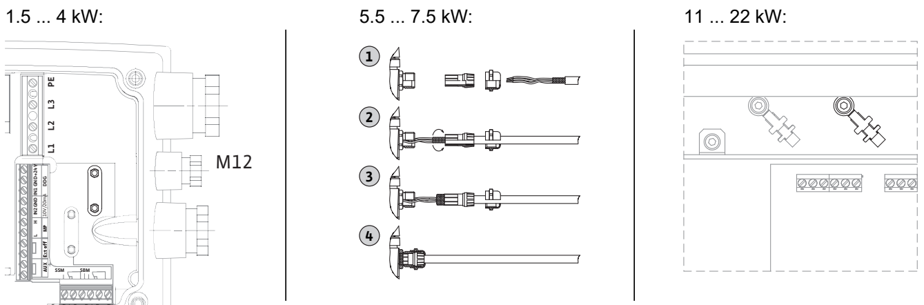
Fig. 25: 连接屏蔽
