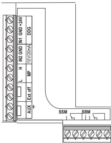
Fig. 26: 控制端子
