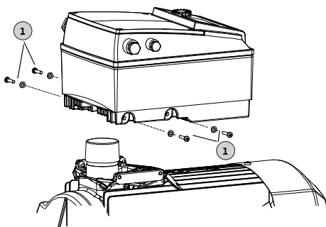
Fig. 49: 电子模块连接 – 电机
