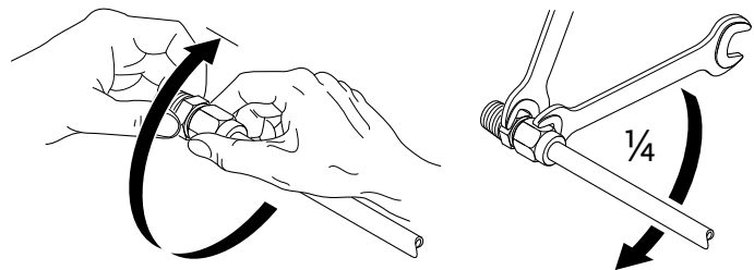
Fig. 19: 将夹紧环螺纹连接再转 1/4 圈
