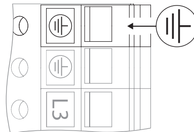
Fig. 28: 额外的接地，11 kW以上的电机
