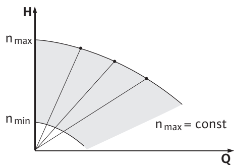
Fig. 8: Varvtalsstyrning
