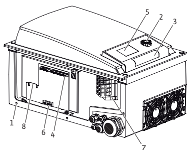
Fig. 5: Elektronikmodul, översikt
