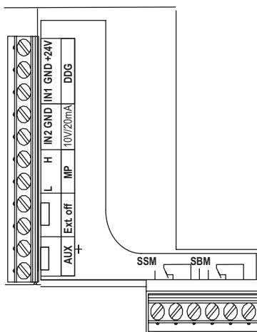
Fig. 26: Styrplintar
