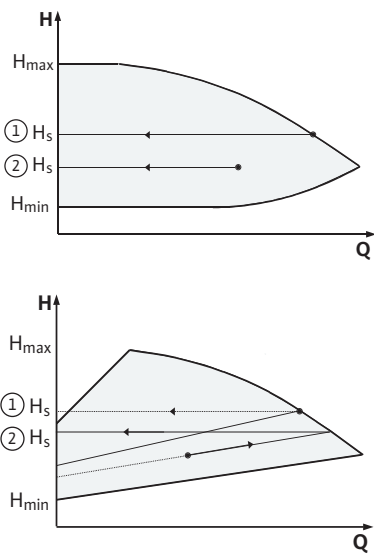
Fig. 32: Reglering Δp-c/Δp-v
