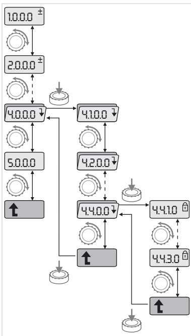
Fig. 43: Navigeringsexempel
