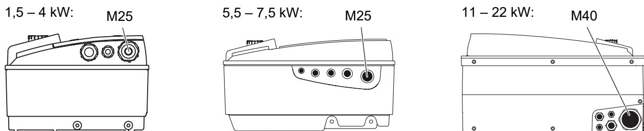
Fig. 24: Kábelcsavarzat a hálózati csatlakozáshoz
