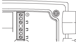
Fig. 27: Teljesítménykapcsok
