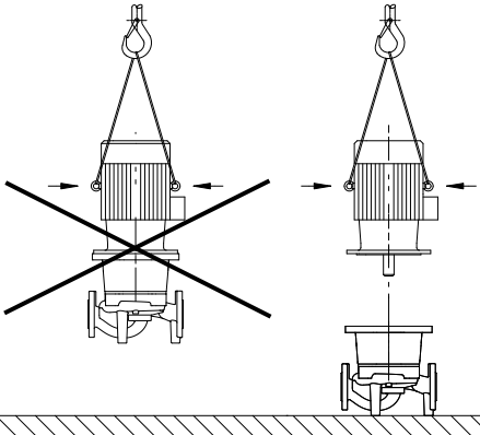
Fig. 2: A motor szállítása
