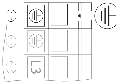
Fig. 28: Kiegészítő földelés, 11 kW motorteljesítménytől
