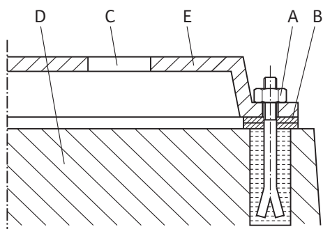
Fig. 16: Példa az alapra történő csavarozásra
