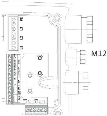
Fig. 25: Árnyékolás csatlakoztatása
