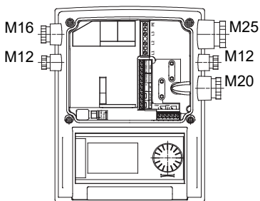
Fig. 29: Kábelcsavarzatok
