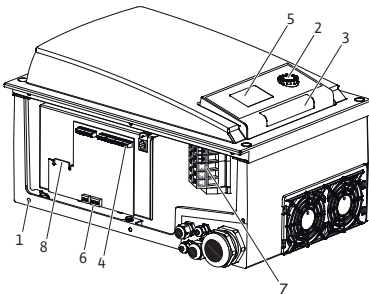
Fig. 5: Elektronikamodul, áttekintés
