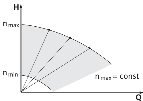
Fig. 33: Állító üzemmód
