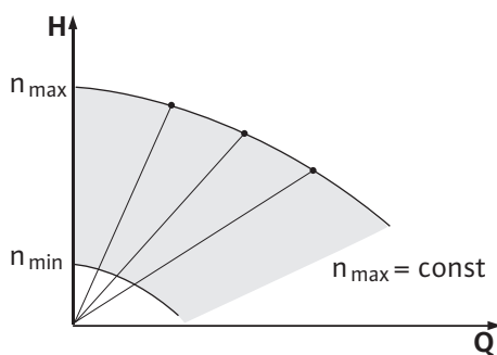
Fig. 8: Állító üzemmód
