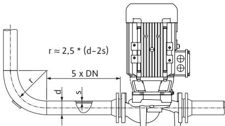
Fig. 18: A szivattyú előtti és utáni csillapítási szakasz
