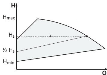
Fig. 7: Szabályzási mód \Delta p -v
