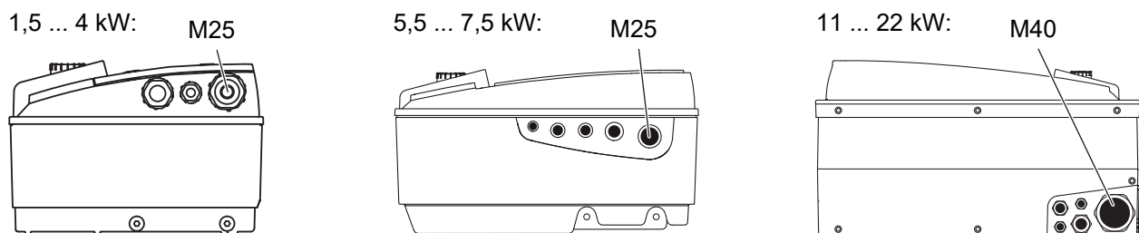
Fig. 24: Maitinimo įtampos kabeliui skirti kabelio priveržikliai
