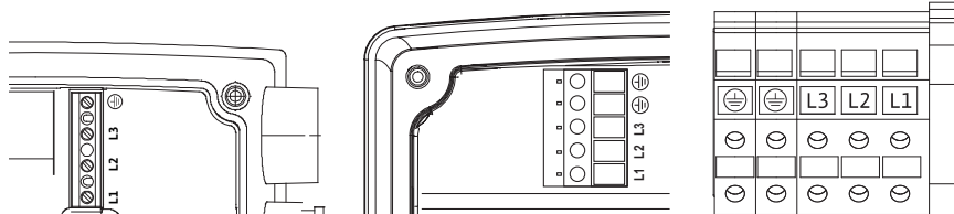
Fig. 27: Elektros gnybtai
