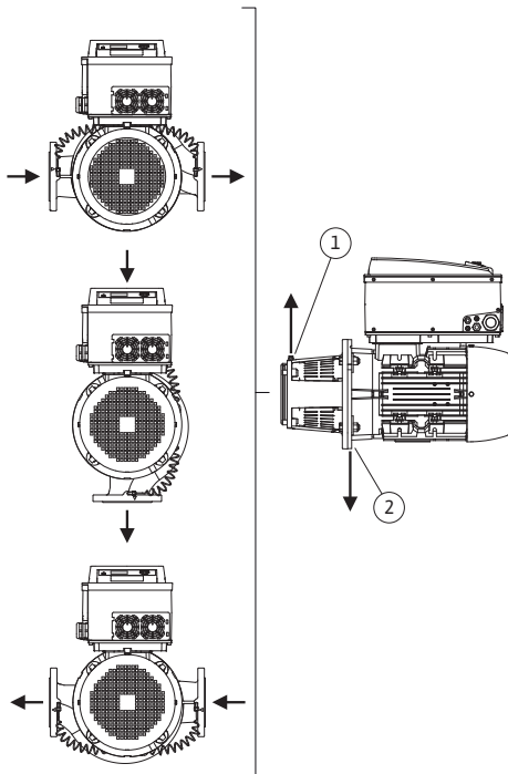
Fig. 14: Leistinos montavimo padėtys su horizontaliu variklio velenu
