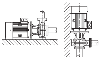
Fig. 4: „Atmos GIGA-B“ vaizdas
