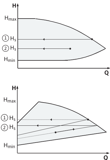
Fig. 32: Reguliavimas Δp-c/Δp-v
