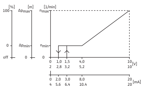
Fig. 12: Начин на функциониране на входовете и изходите
