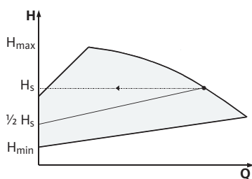
Fig. 7: Режим на регулиране Др-в
