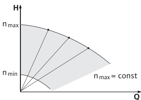
Fig. 33: Режим на управление
