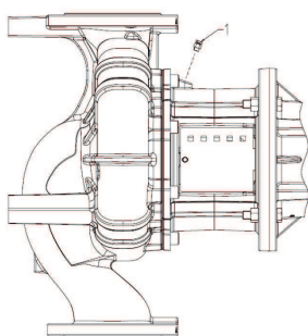
Fig. 30: Обезвъздушителен вентил
