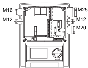
Fig. 29: Кабелни съединения с резба
