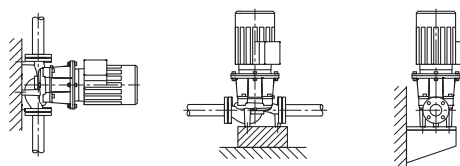
Fig. 3: Weergave IL-E
