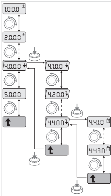
Fig. 43: Navigatievoorbeeld
