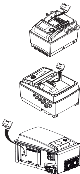
Fig. 10: IF-module aanbrengen
