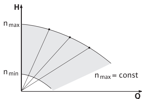
Fig. 33: Regelbedrijf
