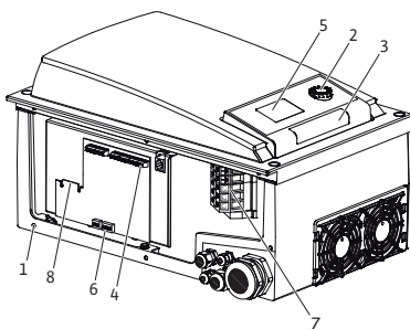
Fig. 5: Elektronica module, overzicht
