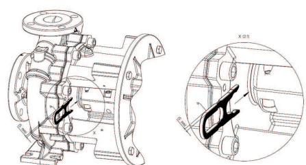
Fig. 47: Aanbrengen van de montagevork
