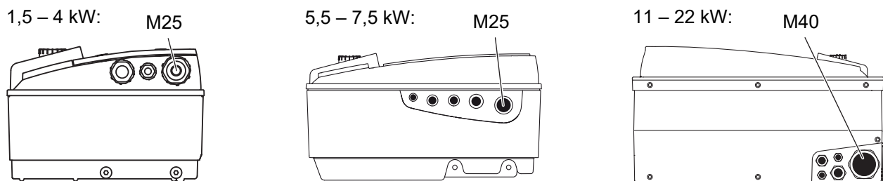
Fig. 24: Kabelschroefverbindingen voor netaansluitleidingen
