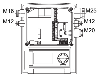
Fig. 29: Kabelschroefverbindingen
