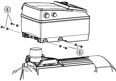
Fig. 48: Elektronik modülün deęiřtirilmesi
