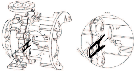
Fig. 47: Montaj çatalının yerleştirilmesi
