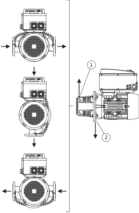
Fig. 14: Yatay motor mili ile izin verilen montaj konumları
