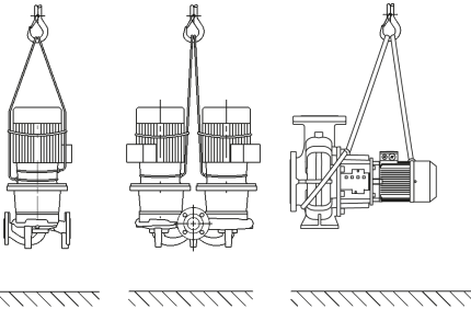
Fig. 1: Pompanın nakliyesi
