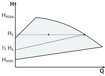
Fig. 7: Kontrol modu Δp-v
