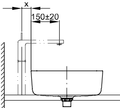
Montage- und Anschlussmaße:
