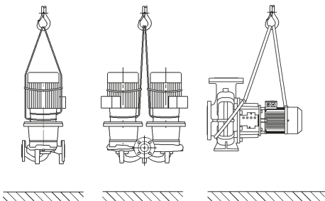
Fig. 1: Pumpun kuljetus
