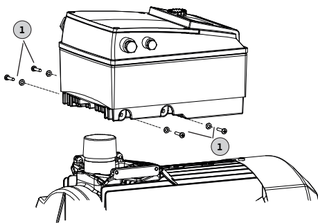
Fig. 48: Elektroniikkamoduulin vaihto
