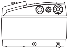
Fig. 24: Verkko-liitäntäjohdon kaapeliläpiviennit
