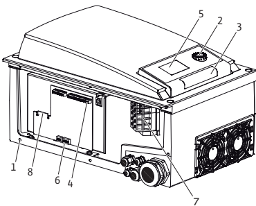
Fig. 5: Elektroniikkamoduuli, yleiskatsaus
