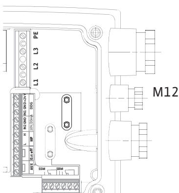
Fig. 25: Suojauksen liittäminen
