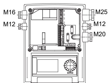
Fig. 29: Kaapeliläpiviennit
