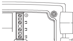
Fig. 27: Teholiittimet
