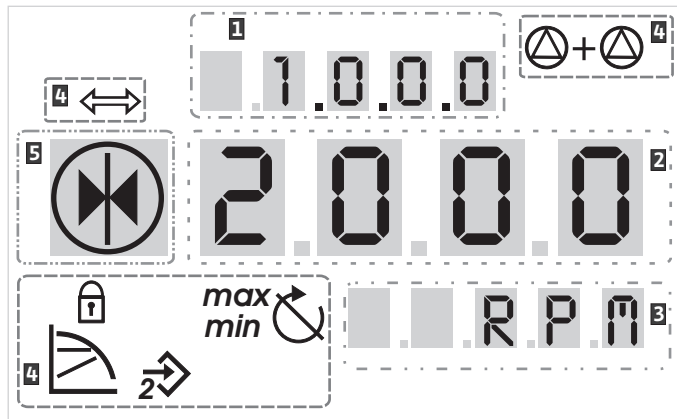
Fig. 36: Näytön rakenne
