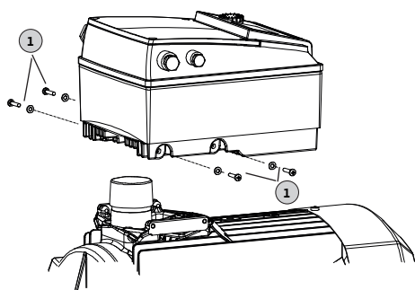
Fig. 48: Αντικατάσταση ηλεκτρονικής μονάδας
