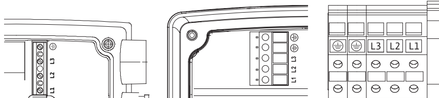
Fig. 27: Ακροδέκτες ισχύος
