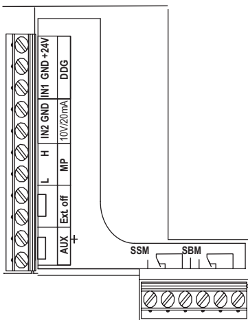
Fig. 26: Ακροδέκτες ελέγχου
