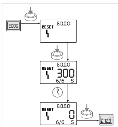
Fig. 56: Ακύρωση σφάλματος τύπου B (X=Y)
