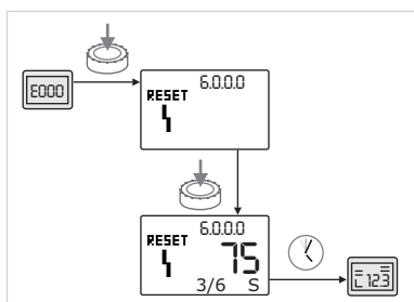
Fig. 55: Ακύρωση σφάλματος τύπου B (X < Y)
