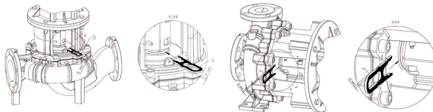
Φουρέτα συναρμολόγησης για εργασίες ρύθμισης
