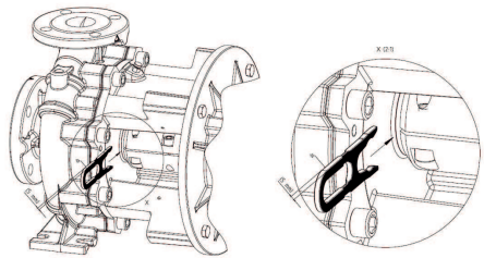
Fig. 47: Τοποθέτηση της φουρκέτας συναρμολόγησης
