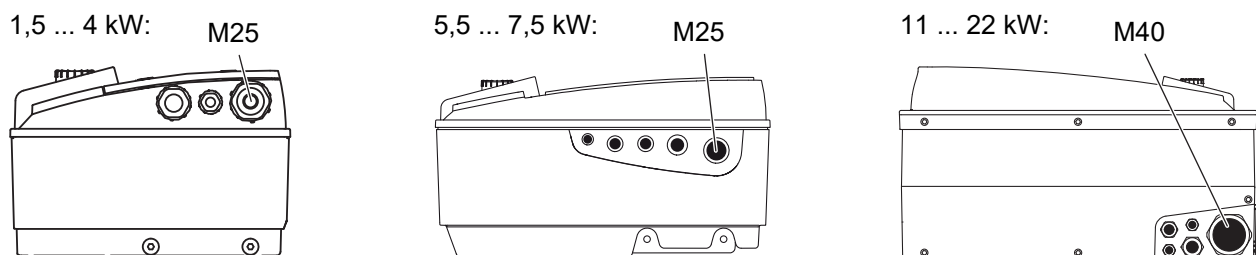
Fig. 24: Στυπιοθλιπτες καλωδίου για καλώδιο ηλεκτρικής σύνδεσης
