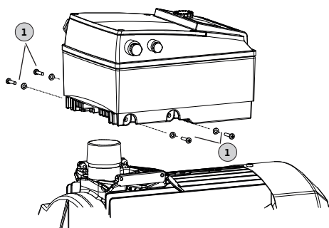
Fig. 49: Σύνδεση ηλεκτρονική μονάδα - κινητήρας
