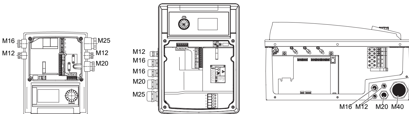
Fig. 29: Στυπιοθλίπτες καλωδίων
