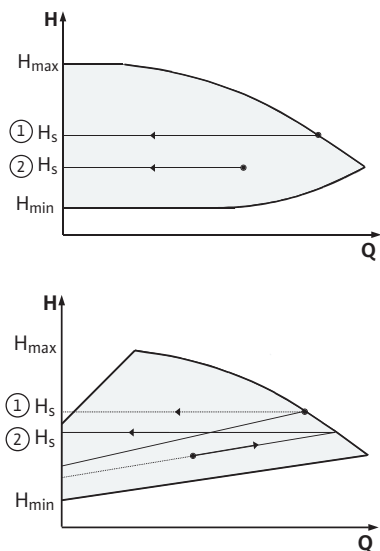
Fig. 32: Σύστημα ρύθμισης Δp-c/Δp-v
