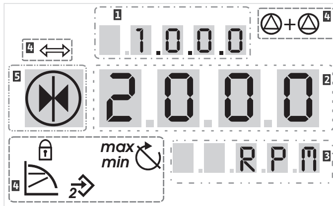
Fig. 36: Structura display-ului
