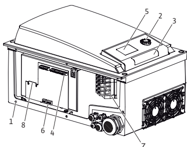
Fig. 5: Presentare generală a modului electronic
