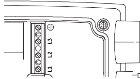
Fig. 27: Borne de putere
