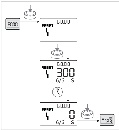
Fig. 56: Квитування помилок типу В (X = Y)
