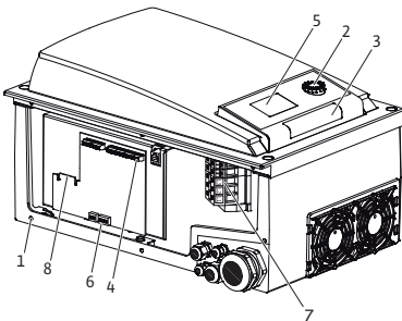
Fig. 5: Електронний модуль, огляд
