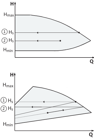
Fig. 32: Регулювання Др-с/Др-в
