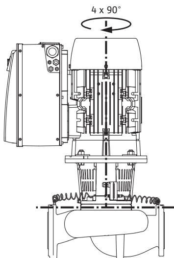
Fig. 17: Прийнятні монтажні положення з вертикальним розташуванням вала двигуна
