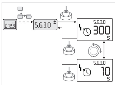
Fig. 44: Налаштування з поверненням до елементу меню «Вибір/налаштування»
