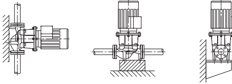
Fig. 3: Виділя IL-E
