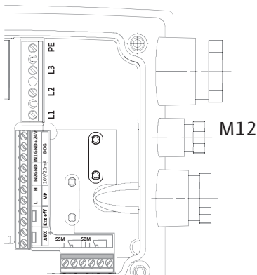
Fig. 25: Під'єднання екрана
