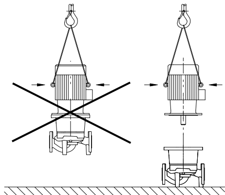
Fig. 2: Транспортування двигуна
