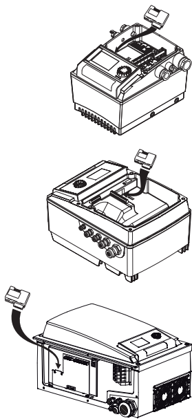
Fig. 10: Застосування IF-модуля
