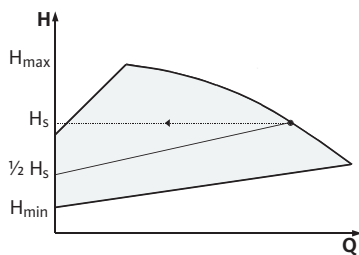
Fig. 7: Спосіб керування \Delta p-v
