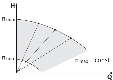
Fig. 8: Режим керування
