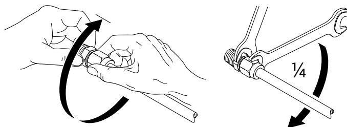
Fig. 19: Повертання затискного різьбового кільця ще на 1/4 оберту
