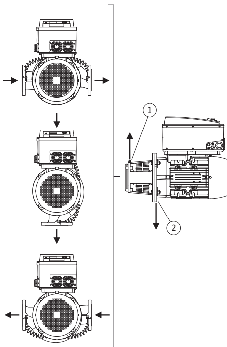
Fig. 14: Прийнятні монтажні положення з горизонтальним розташуванням вала двигуна
