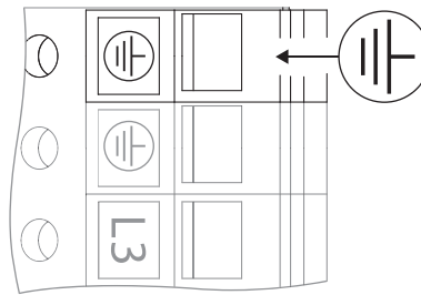
Fig. 28: Додаткове заземлення, потужність двигуна від 11 кВт
