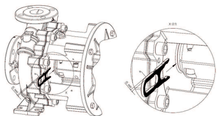
Fig. 47: Встановлення монтажної вилки
