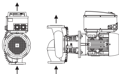
Fig. 13: Розташування компонентів у стані постачання
