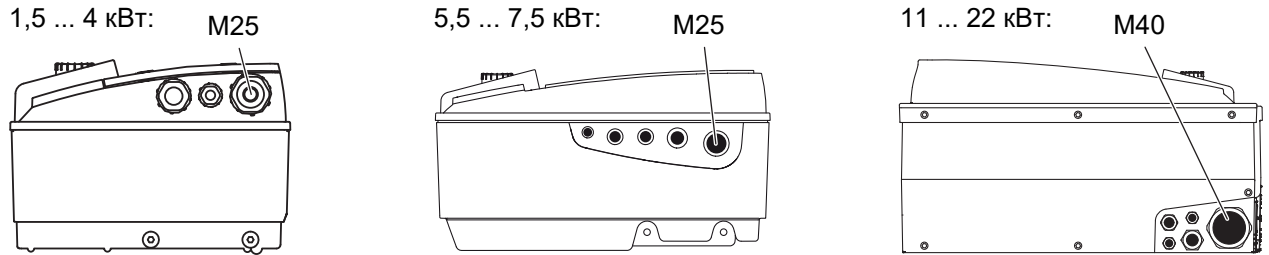
Fig. 24: Кабельні нарізні з'єднання для кабелю під'єднання до мережі
