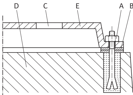
Fig. 16: Приклад гвинтового з'єднання з фундаментом
