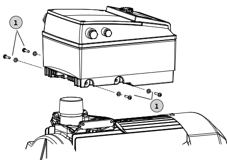
Fig. 48: Заміна електронного модуля
