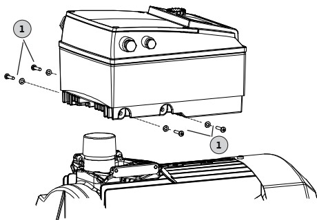
Fig. 49: З'єднання електронного модуля з двигуном
