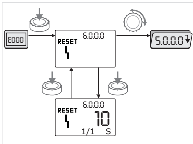
Fig. 50: Навігація в разі помилки
