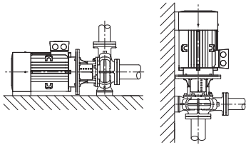
Fig. 4: Вид Atmos GIGA-B
