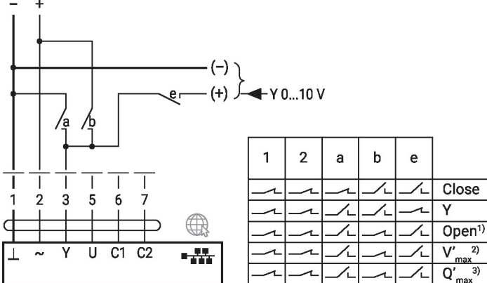
Dwangsturing en -begrenzing met AC 24 V met relaiscontacten (met conventionele besturing of hybride modus)
