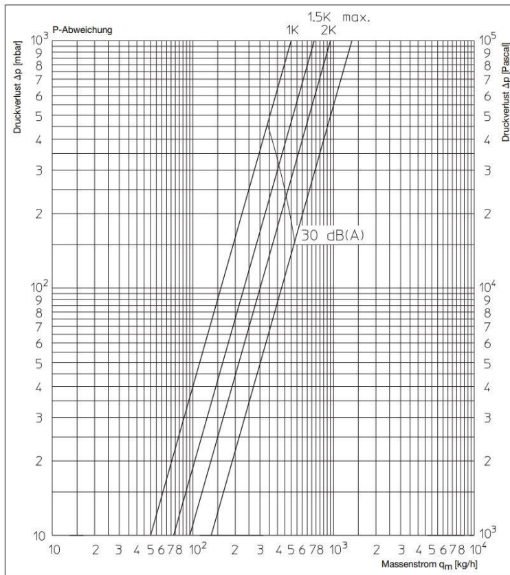
Diagramm 1 Oventrop Thermostatventile „A“ und „RF“, DN 10 und DN 15 Alle Ausführungen 1 bis 2 K P-Abweichung und K_{VS}
