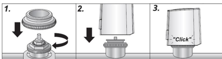
Figuur 1: Montage stelaandrijving
