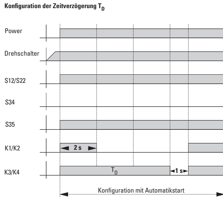
Abbildung 5: Konfiguration der Zeitverzögerung
