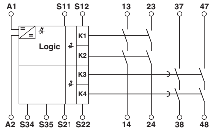
Abbildung 2: Blockschaltbild
