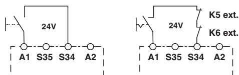
Abbildung 15: Manueller Startkreis
