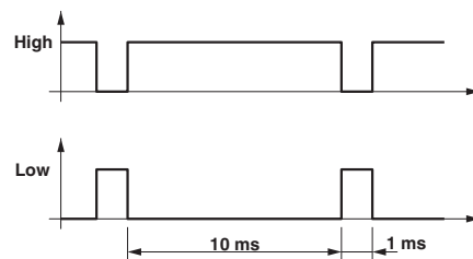
Abbildung 11: Erlaubte Signalform für Lichtgitter, Safe-SPS/PLC und API-Safe
