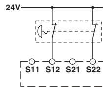
Abbildung 12: Zweikanalig ohne Querschchlussüberwachung
