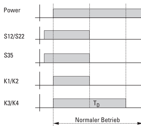
Abbildung 7: Automatischer Reset
