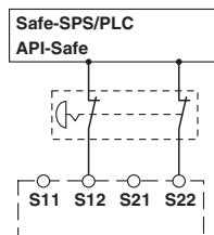
Abbildung 10: Querschchlussüberwachung über externe Taktsignale
