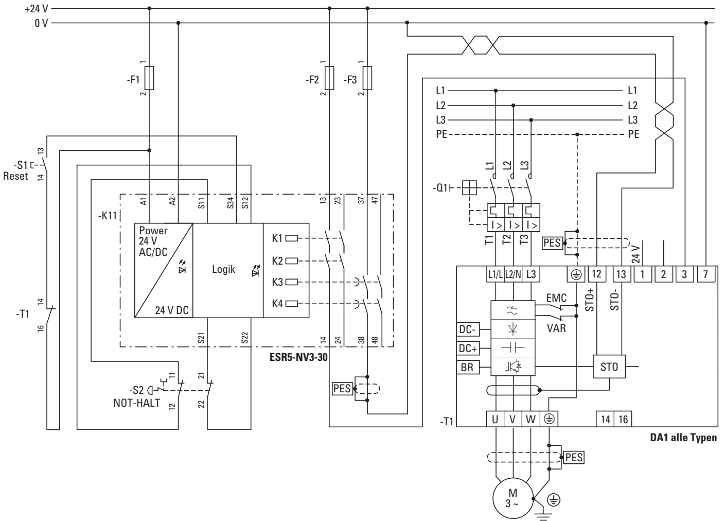
Abbildung 16: Zweikanalige NOT-HALT-Schaltung über STO am Frequenzumrichter DA1
