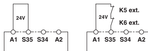
Abbildung 14: Automatischer Startkreis
