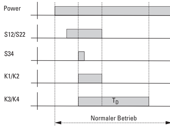
Abbildung 6: Manueller, überwachter Reset
