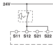
Abbildung 13: Einkanalig ohne Querschlusserkennung
