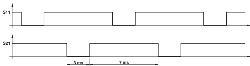
Abbildung 9: Signalform der Taktausgänge
