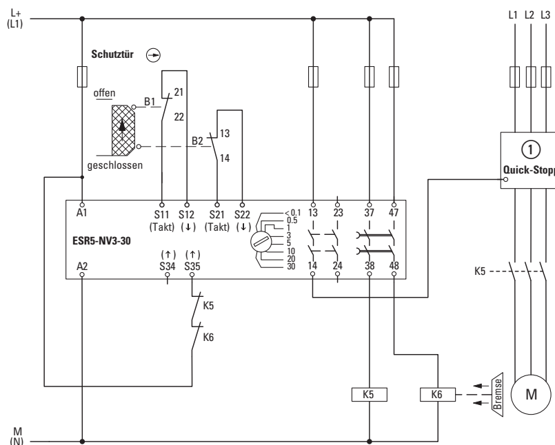
Abbildung 17: Zweikanalige Schutztürüberwachung mit abfallverzögerten Kontakten und automatischem Reset
