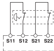
Abbildung 8: Querschchlussüberwachung
