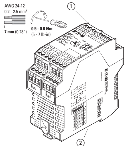
Abbildung 1: ESR5-NV3-300 ① Steckbare Schraubklemme COMBICON ② Metallschloss zur Befestigung auf der Tragschiene
