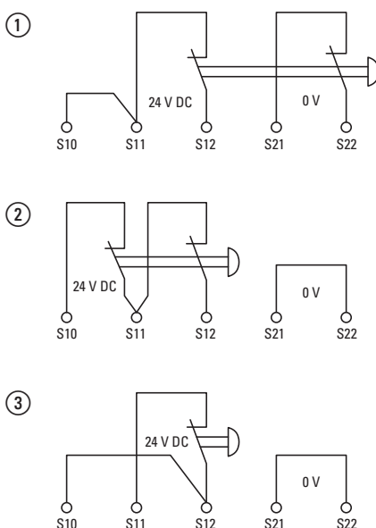
Abbildung 10: Anschlussvarianten Signalgeber
