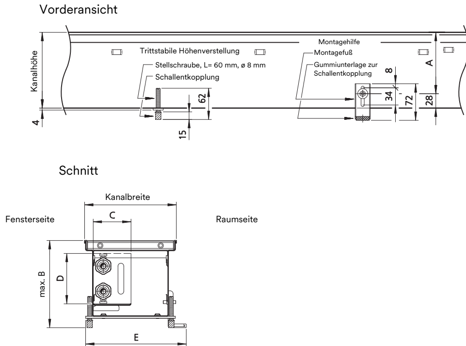
Abb. 3: Höhenverstellung Abmessungen
