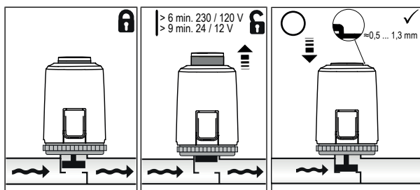
Abb. 1: "First-Open"-Funktion
