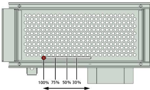
Abb. 4: SchieberEinstellung
