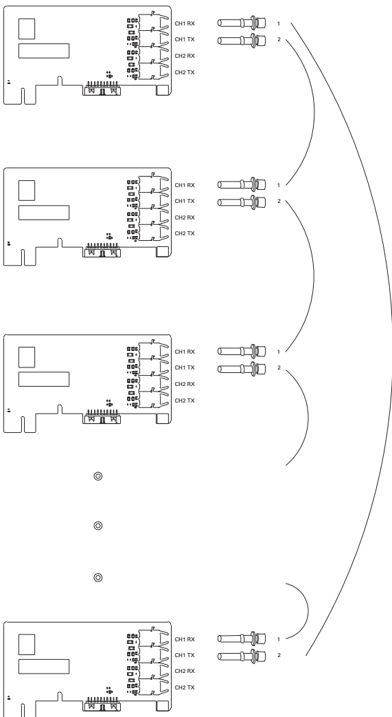
Abbildung 5. Zwei oder mehr PowerXL DX1 Frequenzumrichter-Systeme
