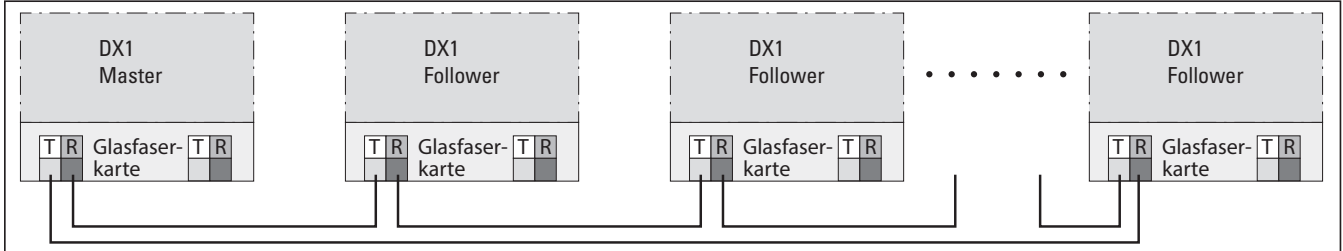
Abbildung 4. Glasfaserkarten-Anschluss für Master-Follower-Konfigurationen
