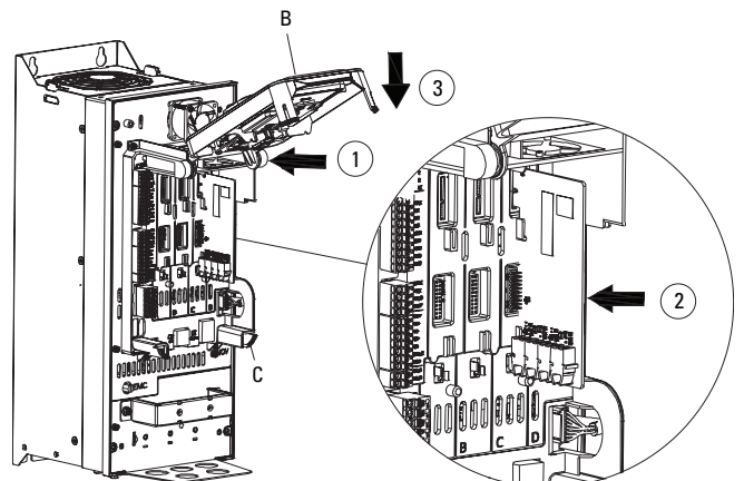
Abbildung 3. Montage der Optionskarten
