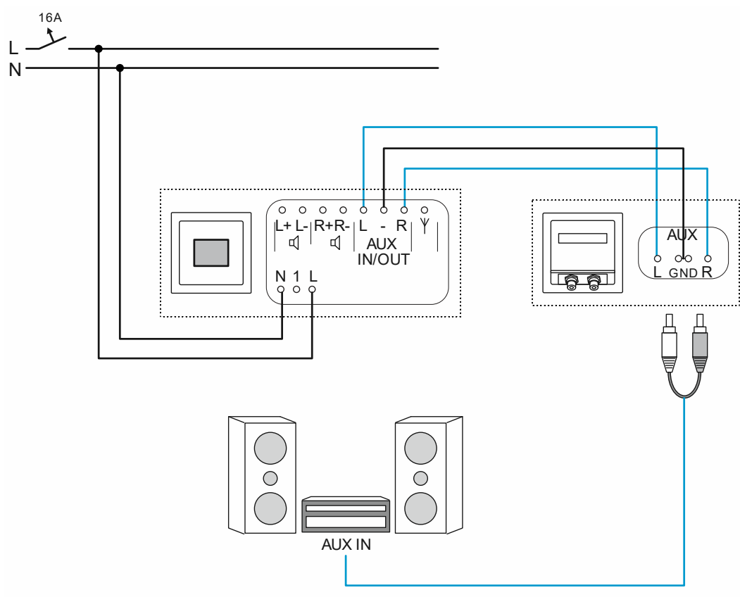
Abb. 91: Unterputz-Radio mit HiFi-Anlage: Übersicht
