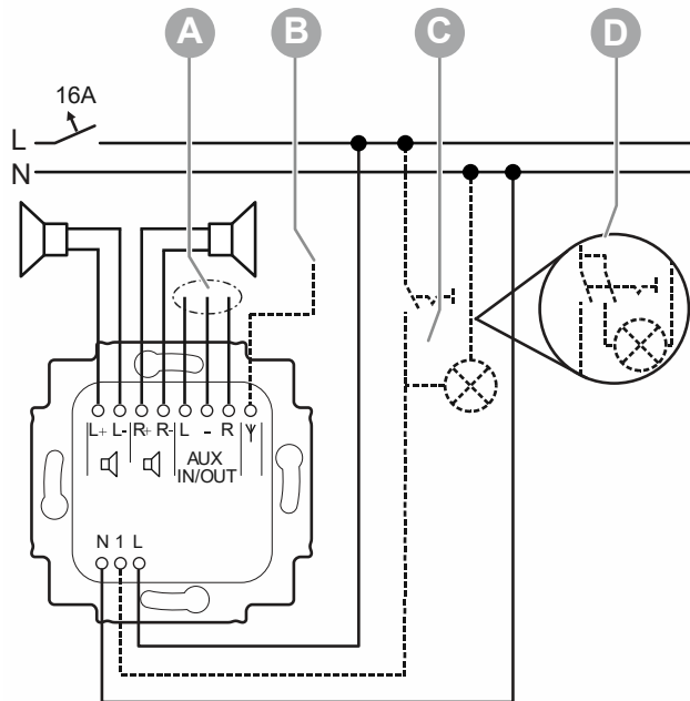
Abb. 8: Elektrischer Anschluss
