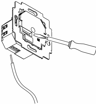
Abb. 4: Netzkabel anschließen
