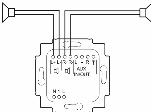
Abb. 10: Lautsprecheranschluss STEREO
