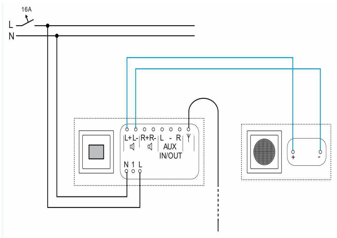
Abb. 79: Einbauset Anschluss (Wurfantenne, ca. 90 cm lang)
