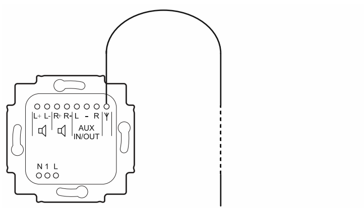
Obr. 14: Anténa
