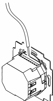
Obr. 3: Připojení kabelů reproduktorů / signálních vedení
