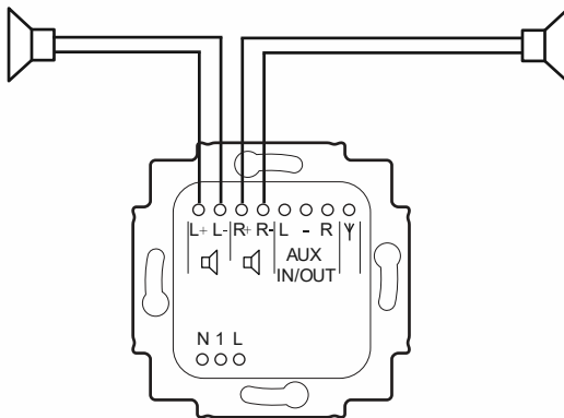
Fig. 10: Conexión de altavoz ESTÉREO
