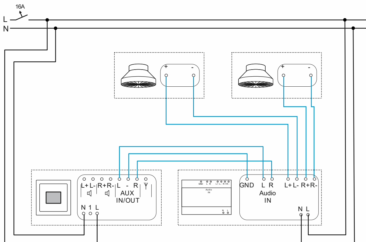
Fig. 90: Radio empotrada con amplificador y 2 altavoces de techo: conexión
