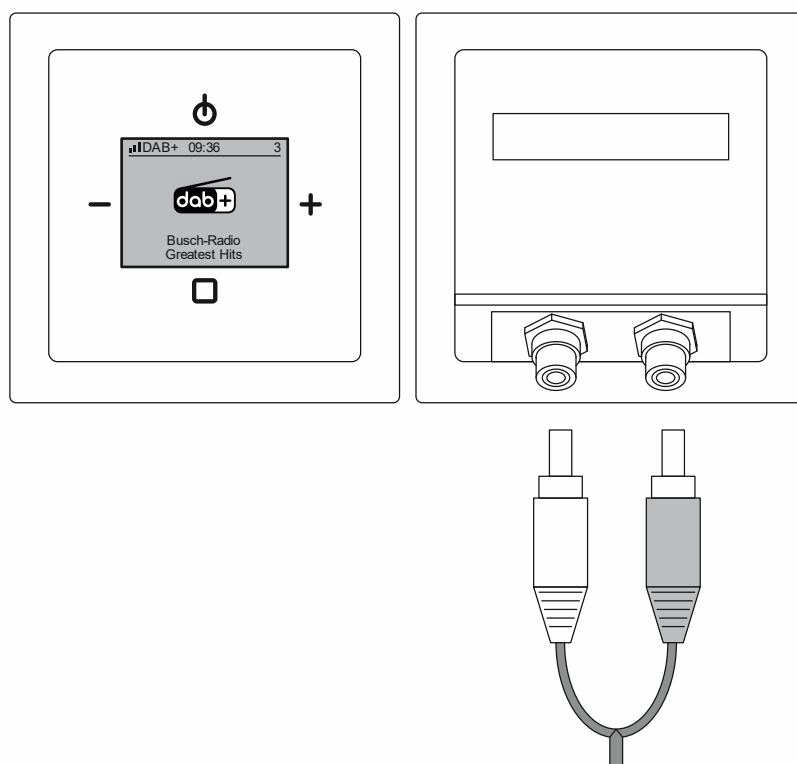
Fig. 13: Extensión AUX cinch
