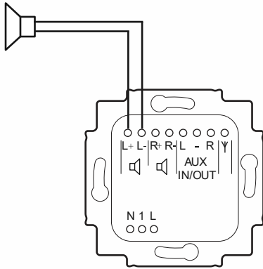
Fig. 9: Conexión de altavoz MONO
