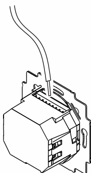
Rys. 3: Podłączanie głośników / przewodów sygnałowych
