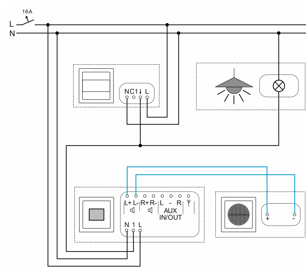
Rys. 83: Zestaw do zabudowy i czujnik ruchu: przyłącze
