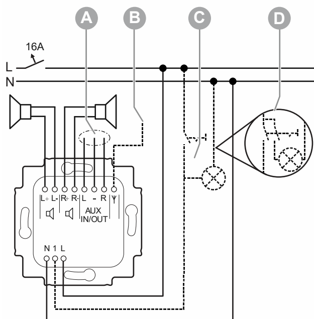
Rys. 8: Przyłącze elektryczne
