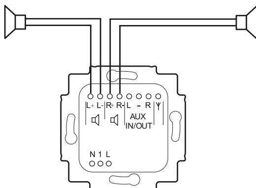
Rys. 10: Podłączanie głośnika STEREO
