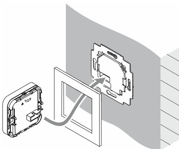
Rys. 6: Montaż wyświetlacza
