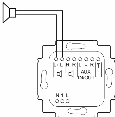
Rys. 9: Podłączanie głośnika MONO
