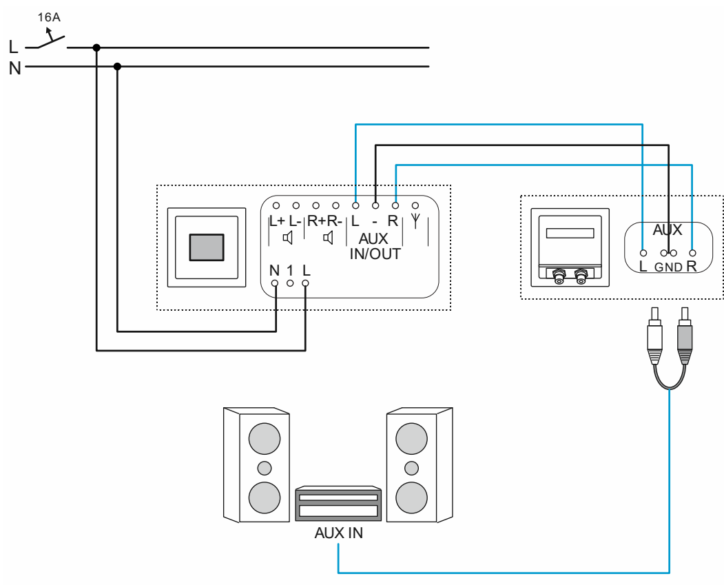
Rys. 92: Radio podtynkowe z systemem hi-fi: podłączenie
