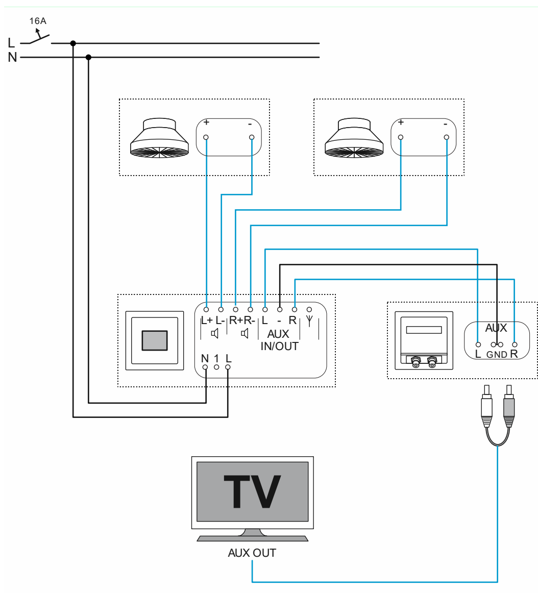
Rys. 96: Radio podtynkowe z TV: podłączenie
