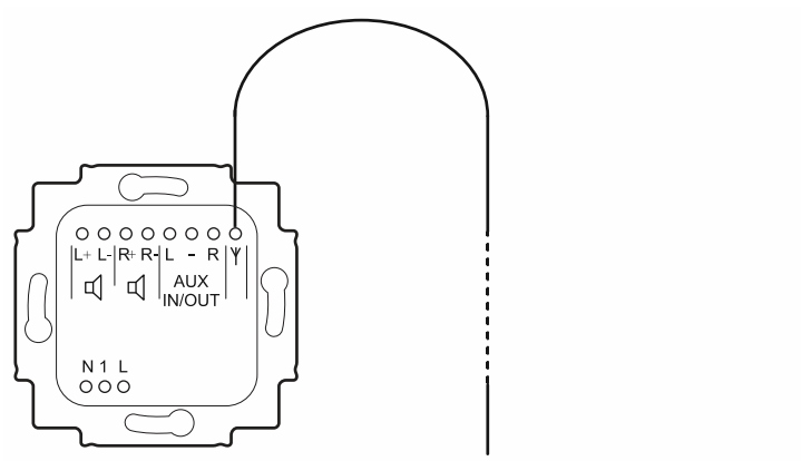
Fig. 14: Antenna
